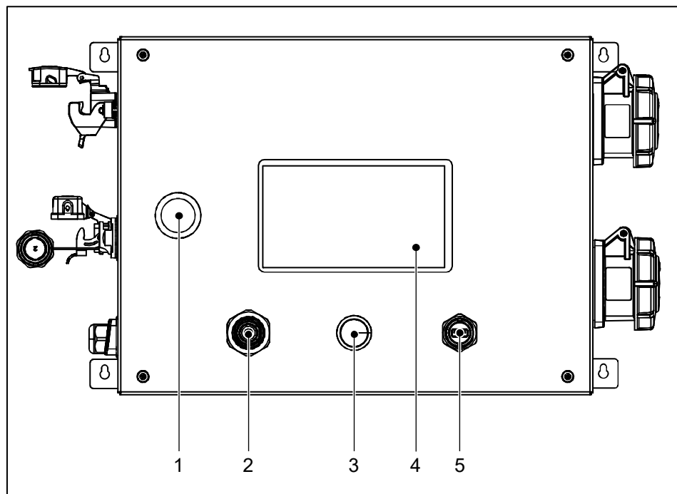
Abb. 3-3 Funktionselemente
