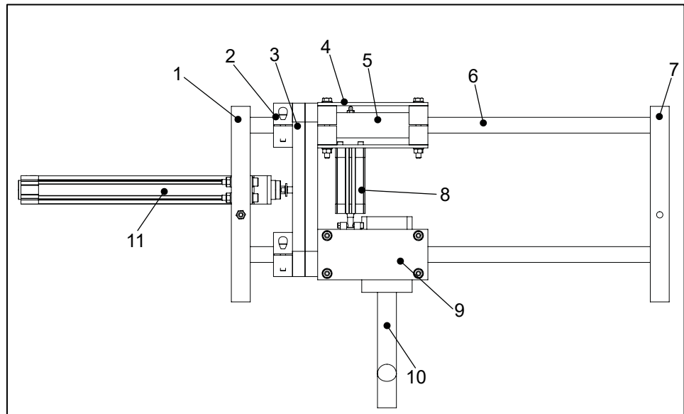
Abb. 3-21 Frontansicht
