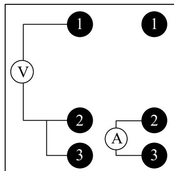
Abb. 8-2 Anschluss Messgerät
