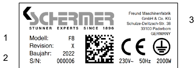
Abb. 3-18 Beispiel Typenschild
