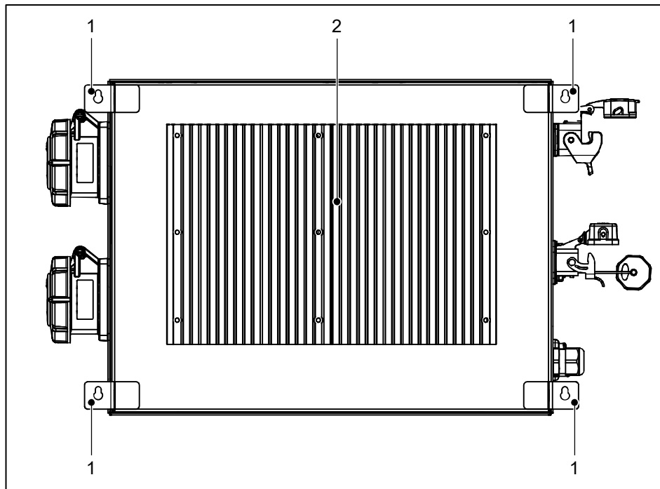
Abb. 3-4 Funktionselemente
