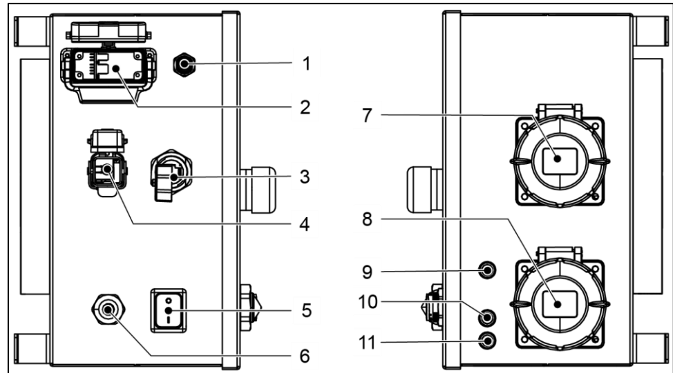
Abb. 3-5 Funktionselemente
