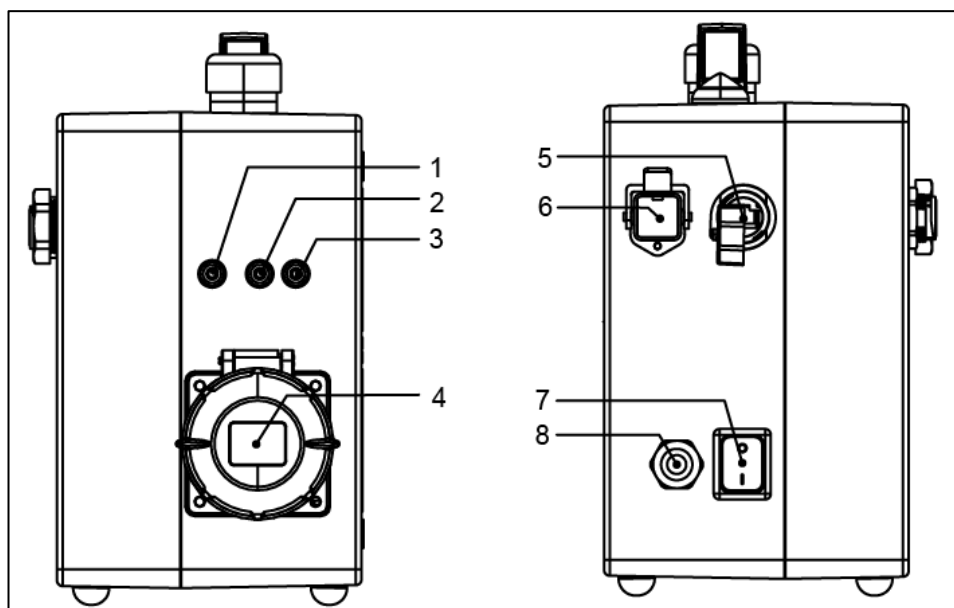
Abb. 3-2 Funktionselemente
