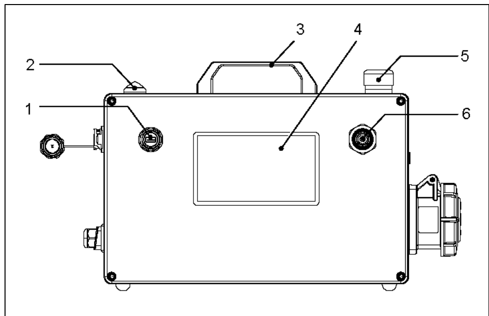
Abb. 3-1 Funktionselemente
