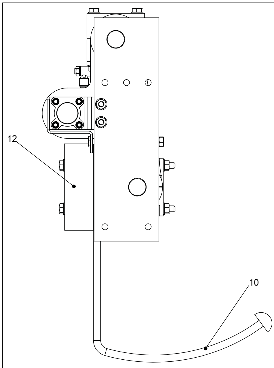
Abb. 3-22 Seitenansicht
