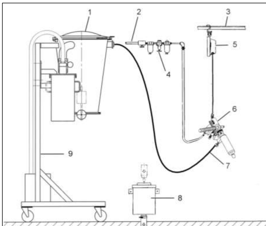
Рис. 3-2 VSS-EDF
