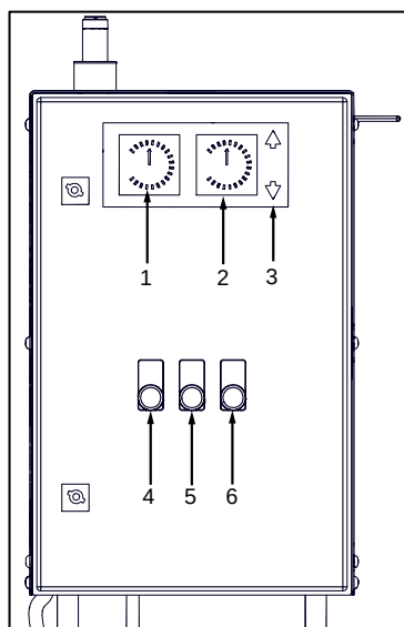
Рис. 3-5 Передняя сторона
