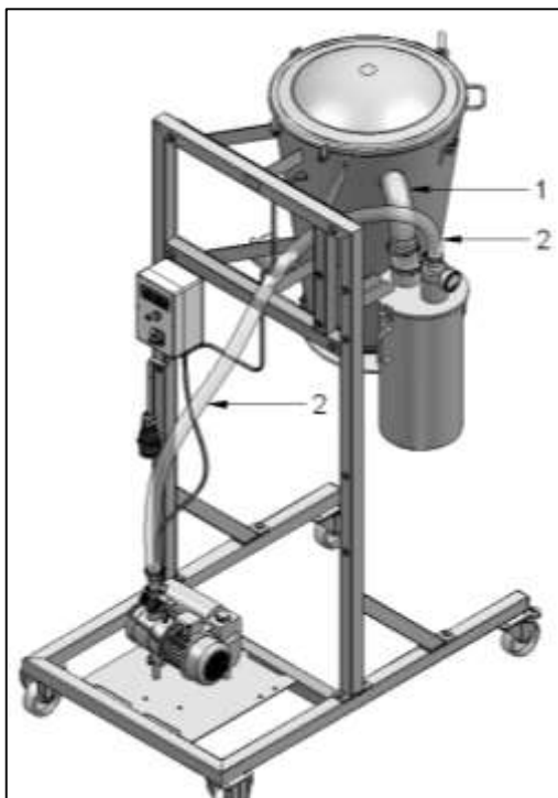
Рис. 6-2 VSS-EDF
