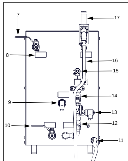
Fig. 3-8 Arrière
