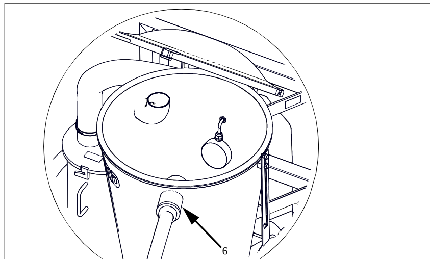
Fig. 6-4 Raccordement tuyau d'aspiration
