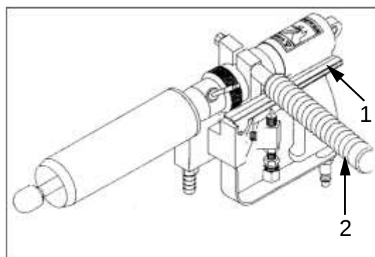
Fig. 7-5 Pièce à main EDF
