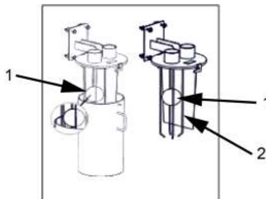
Fig. 3–10 Protección antidesbordamiento del depósito del separador
