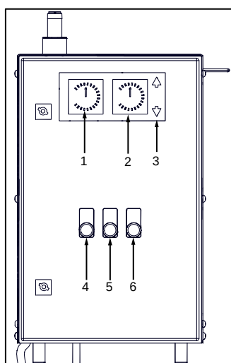
Fig. 3-7 Parte frontal
