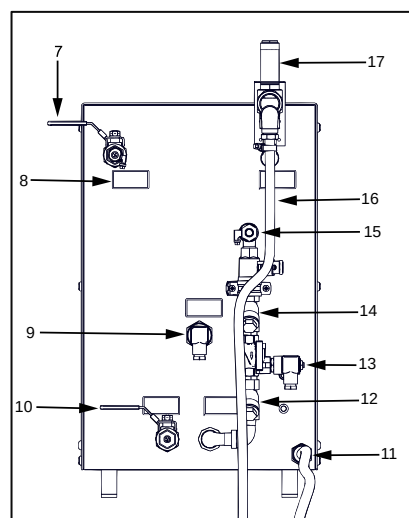
Fig. 3-6 Parte trasera
