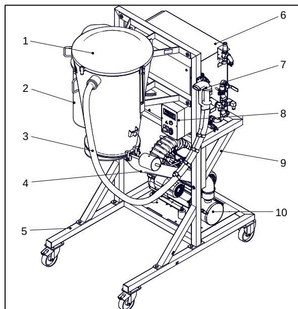
Fig. 3-3 Configuración estándar SVSS
