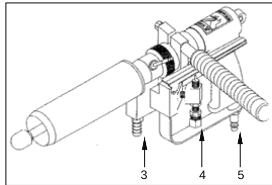
Fig. 6-3 Pieza de mano EDF
