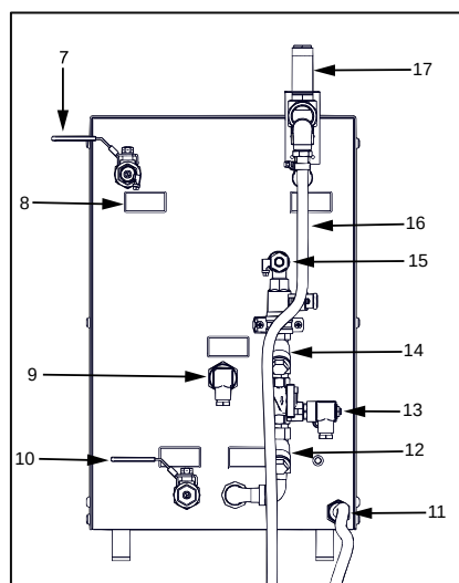
Fig. 7-12 Parte trasera del generador de vapor
