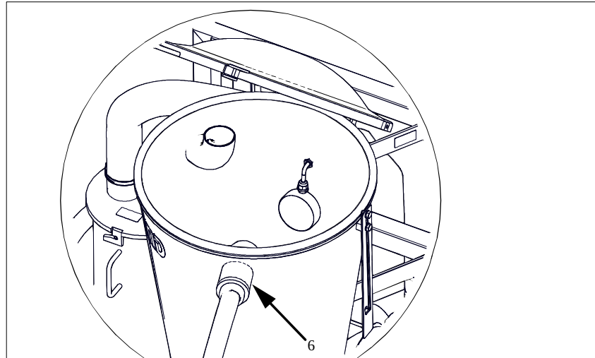
Fig. 6-4 Conexión manguera de aspiración
