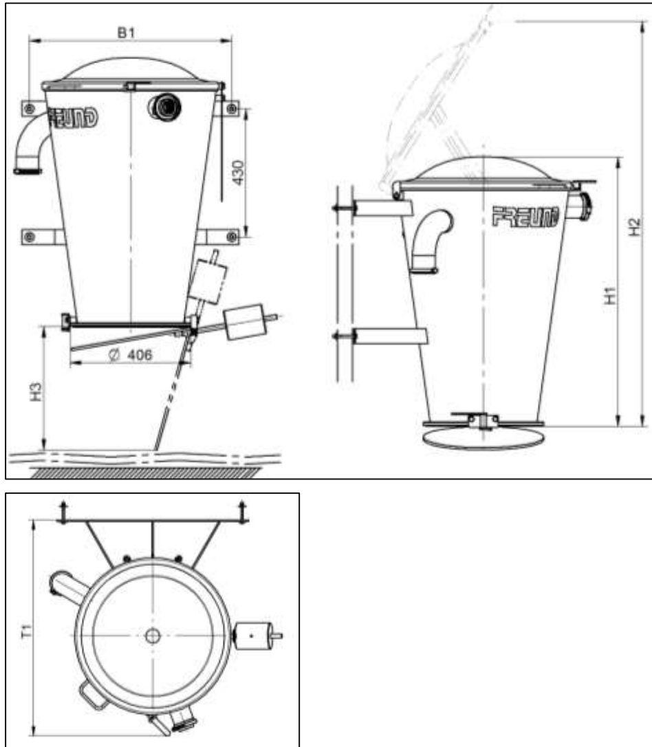
Fig. 3-11 Depósito de vacío
