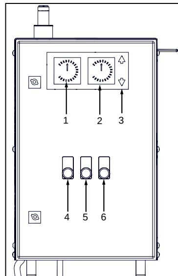
Fig. 3-5 Parte frontal
