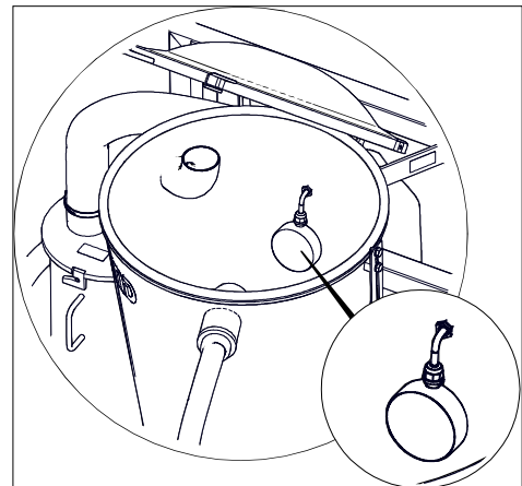
Fig. 3-12 Protección antidesbordamiento del depósito de vacío
