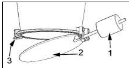
Fig. 7-11 Depósito de vacío con compuerta inferior
