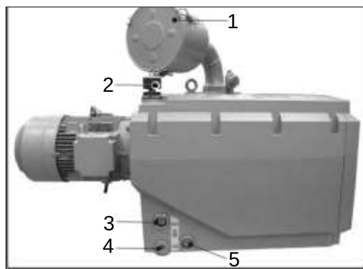
Fig. 9-4 VP100
