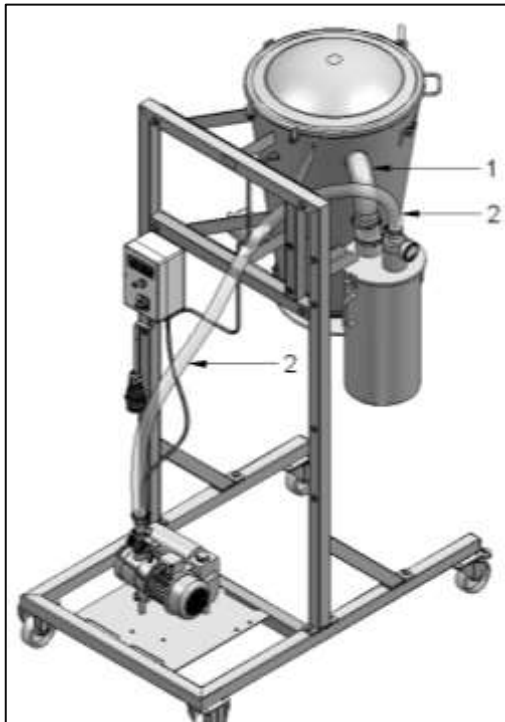
Fig. 6-2 VSS-EDF
