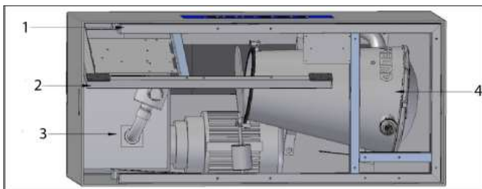
Fig. 5-1 Unidad empaquetada
