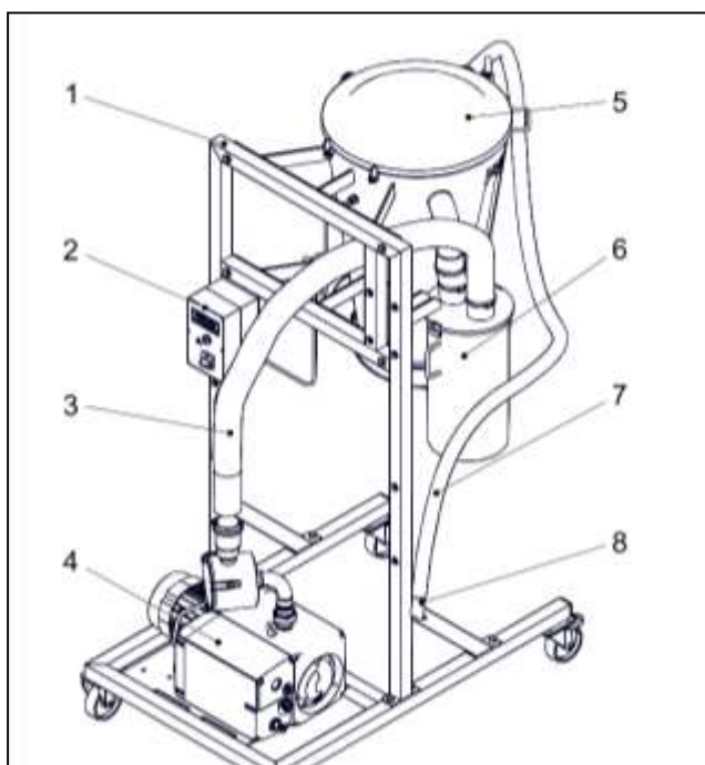
Fig. 3-1 VSS
