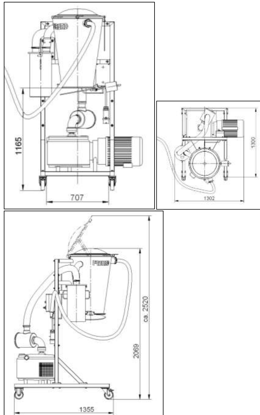
Fig. 3-16 Dimensiones VSS-estándar/VSS-EDF
