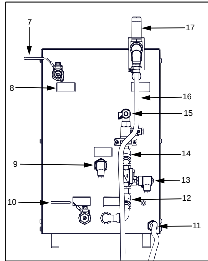
Fig. 7-8 Elementos de mando posteriores
