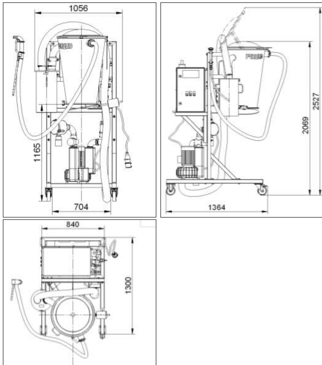
Fig. 3-17 Dimensiones SVSS con carrito
