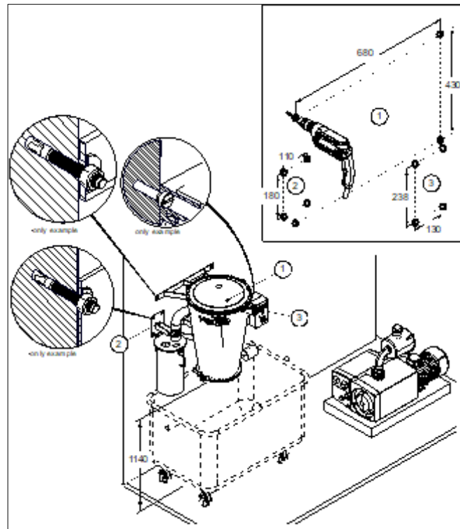
Fig. 3-18 Patrón de agujeros VSS con VT110
