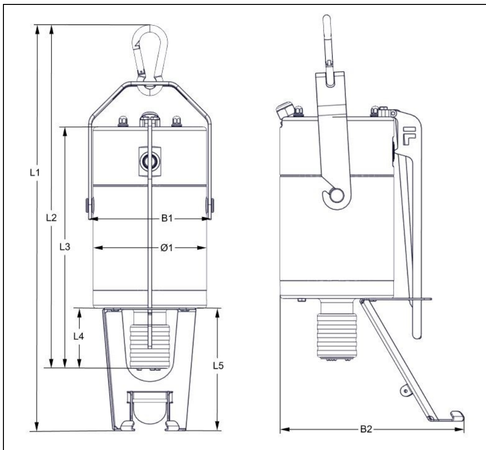
Рис. 3-4 Электродвигатель TM-E6000_evo3
