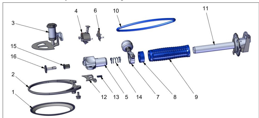
Afb. 3-2 Elektrische trimmer 128_evo3 (voorbeeld)
