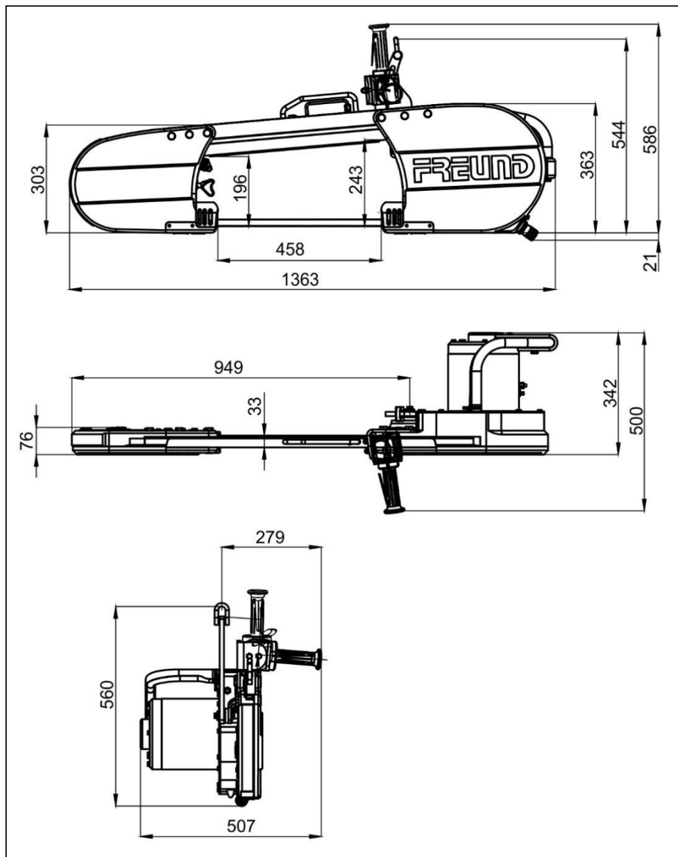
Afb. 3-3 Afmetingen slijtbandzaag (in mm)
