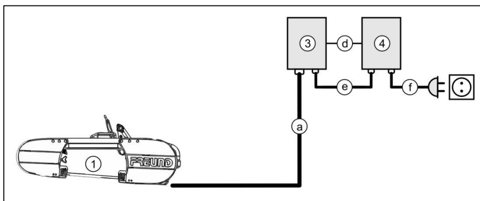
Fig. 5-4 Schéma de raccordement
