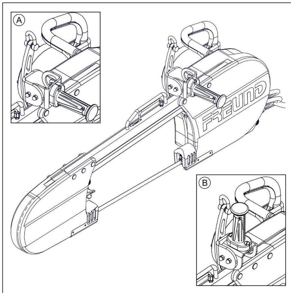
Fig. 3-1 Vue de la SB46-24 avec des détails concernant l'orientation réglable de la poignée (A), (B)
