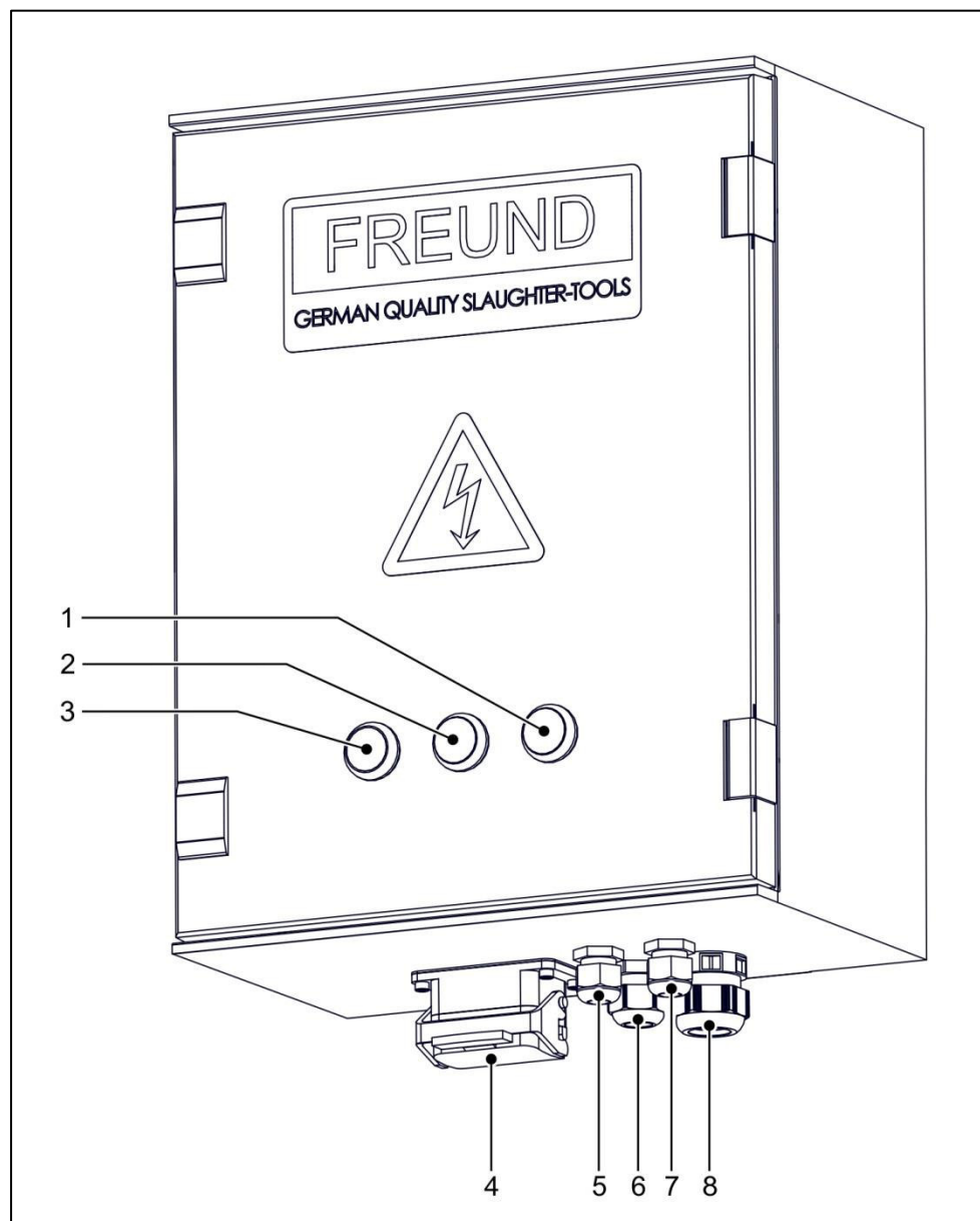
Fig. 3-4 Vue du dispositif de commutation SG SB46-24
