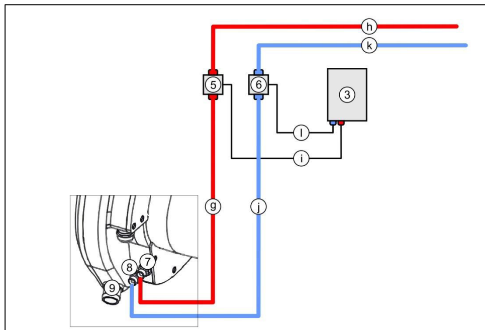
Fig. 5-6 Schéma de raccordement
