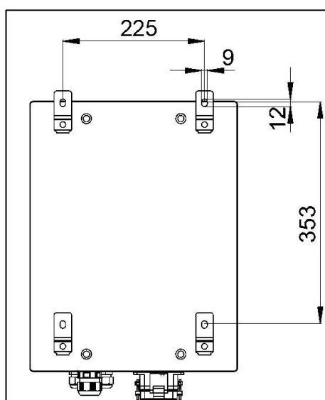
Fig. 5-2 Schéma de perçage du dispositif de commutation [données en mm]
