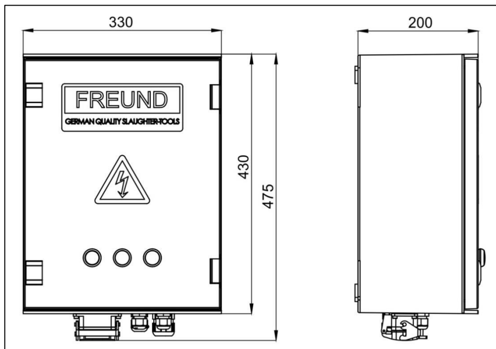
Fig. 3-5 Dimensions du dispositif de commutation (données en mm)
