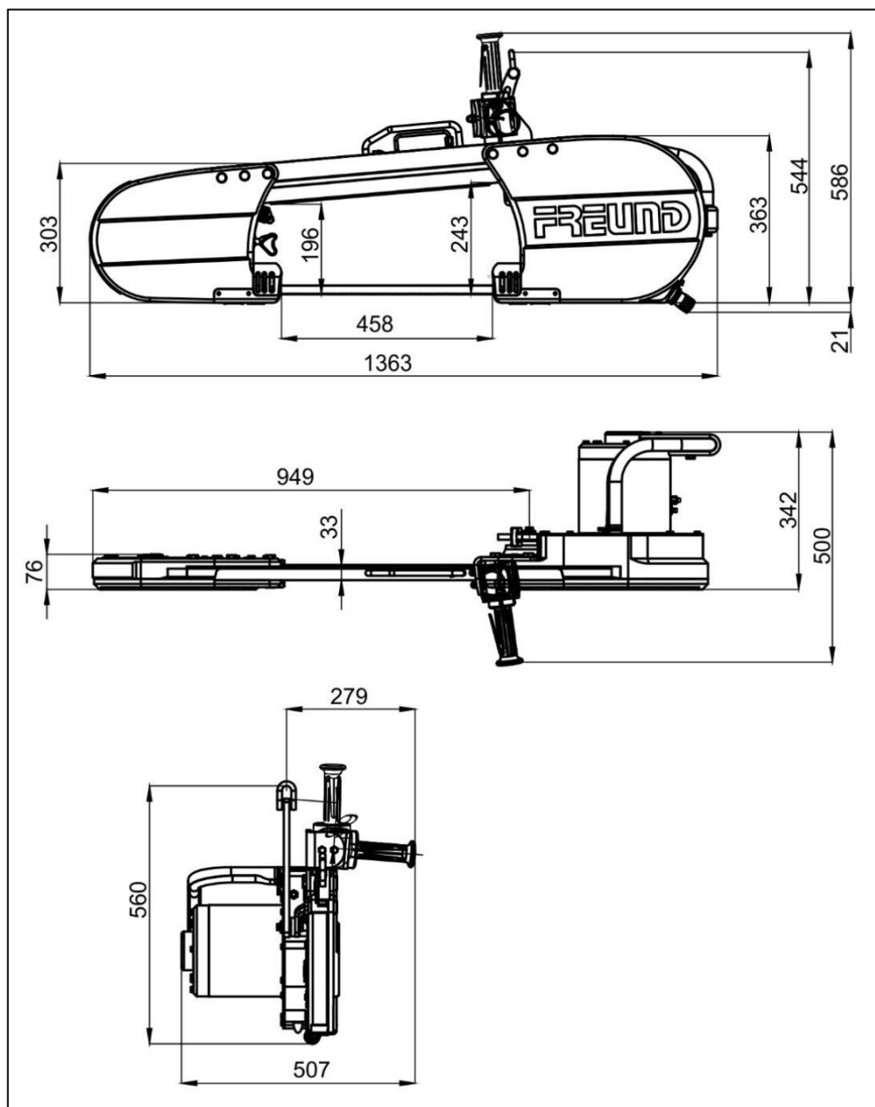
Fig. 3-3 Dimensions de la scie de découpe à ruban (en mm)
