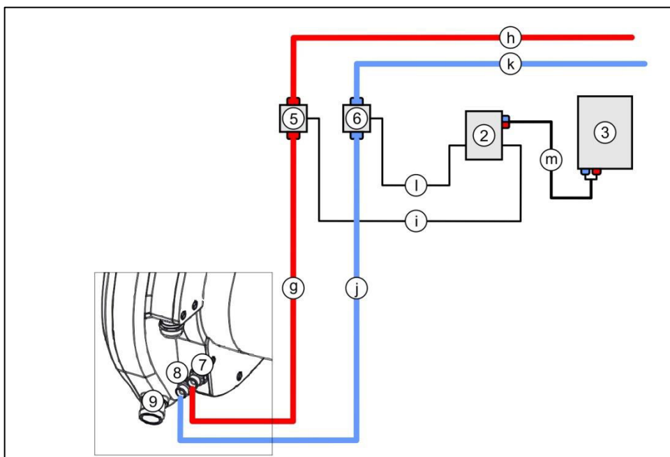
Fig. 5-7 Schéma de raccordement avec boîtier de distribution (option)
