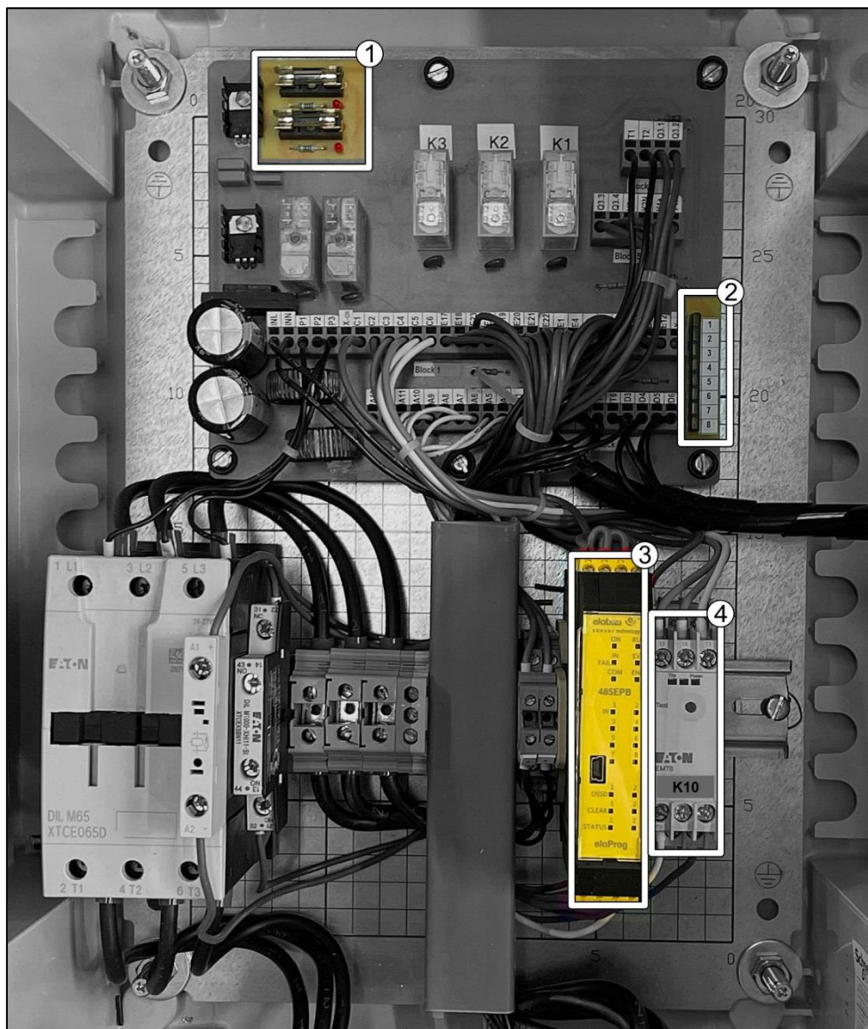
Fig. 9-1 Voyants d'état à LED du dispositif de commutation
