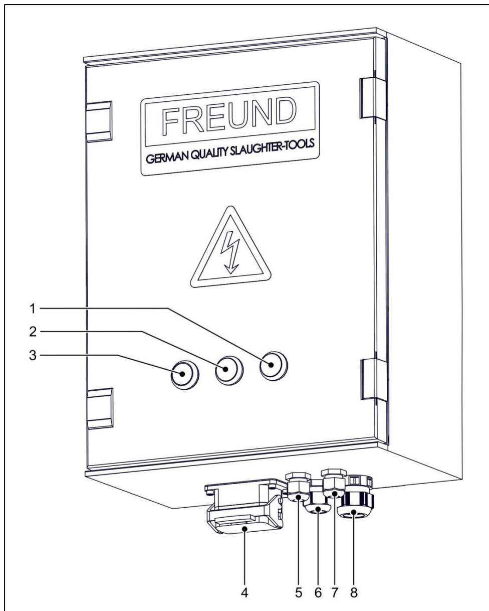
Fig. 3-4 Vista del dispositivo interruptor SG SB46-24
