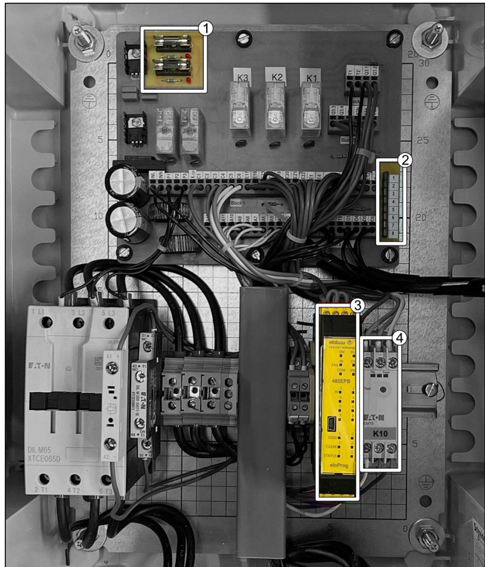
Fig. 9-1 Indicadores de estado LED en el dispositivo interruptor
