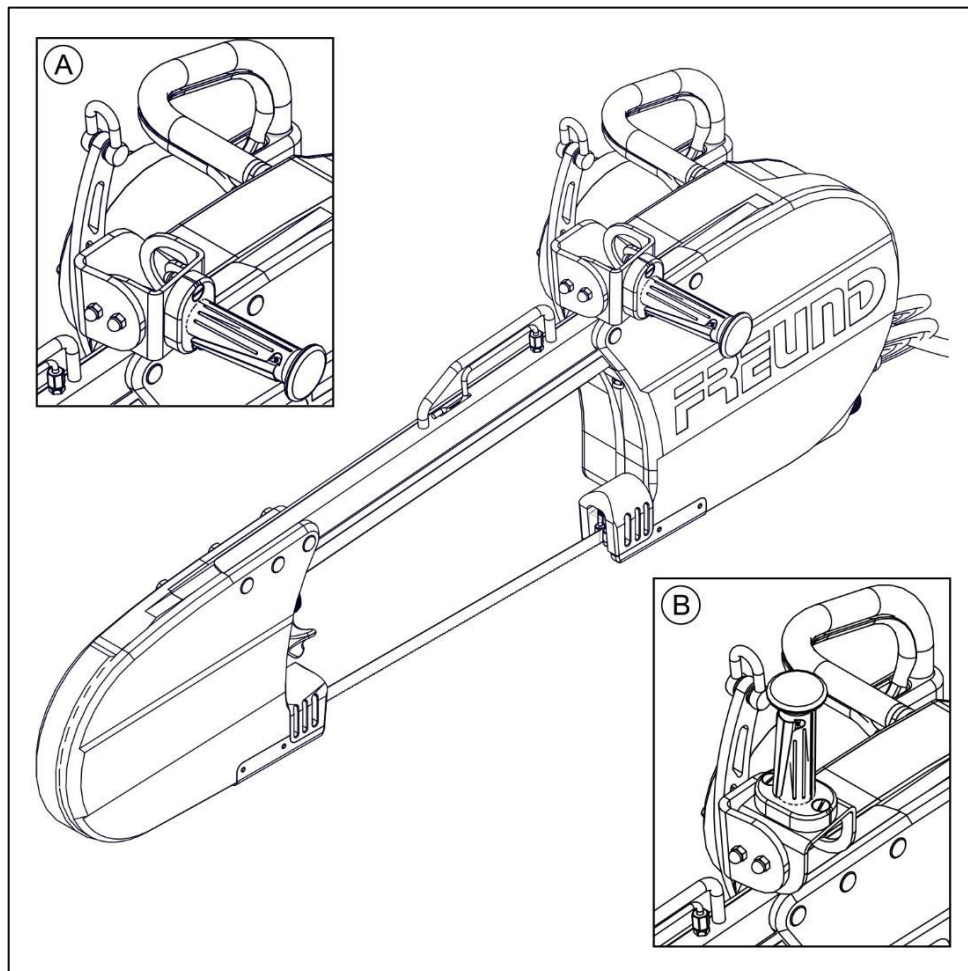
Fig. 3-1 Vista de la SB46-24 con detalles para una orientación ajustable del mango ergonómico (A), (B)
