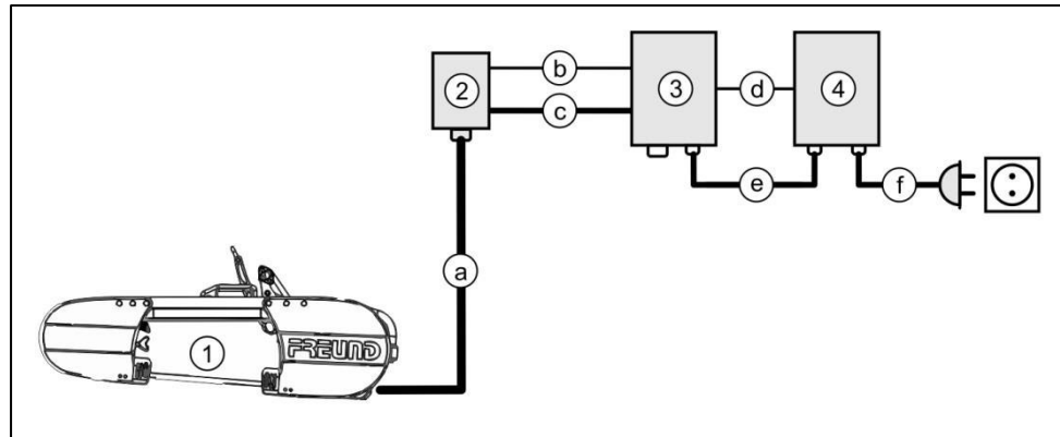
Fig. 5-5 Esquema de conexión con caja de distribución (opcional)
