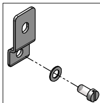
Fig. 5-3 Juego de fijación a pared, opcionalmente disponible, n.º de art. 100-022-069
