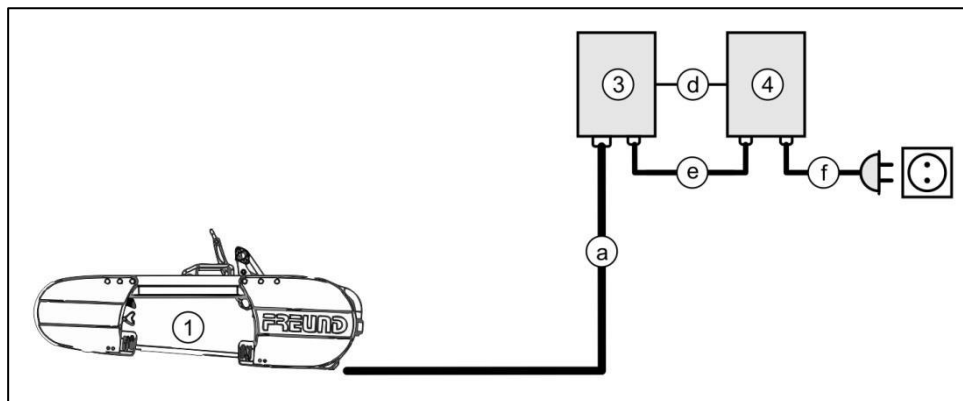
Fig. 5-4 Esquema de conexión
