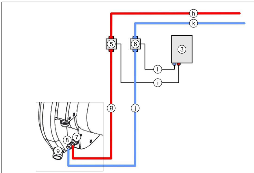
Fig. 5-6 Esquema de conexión
