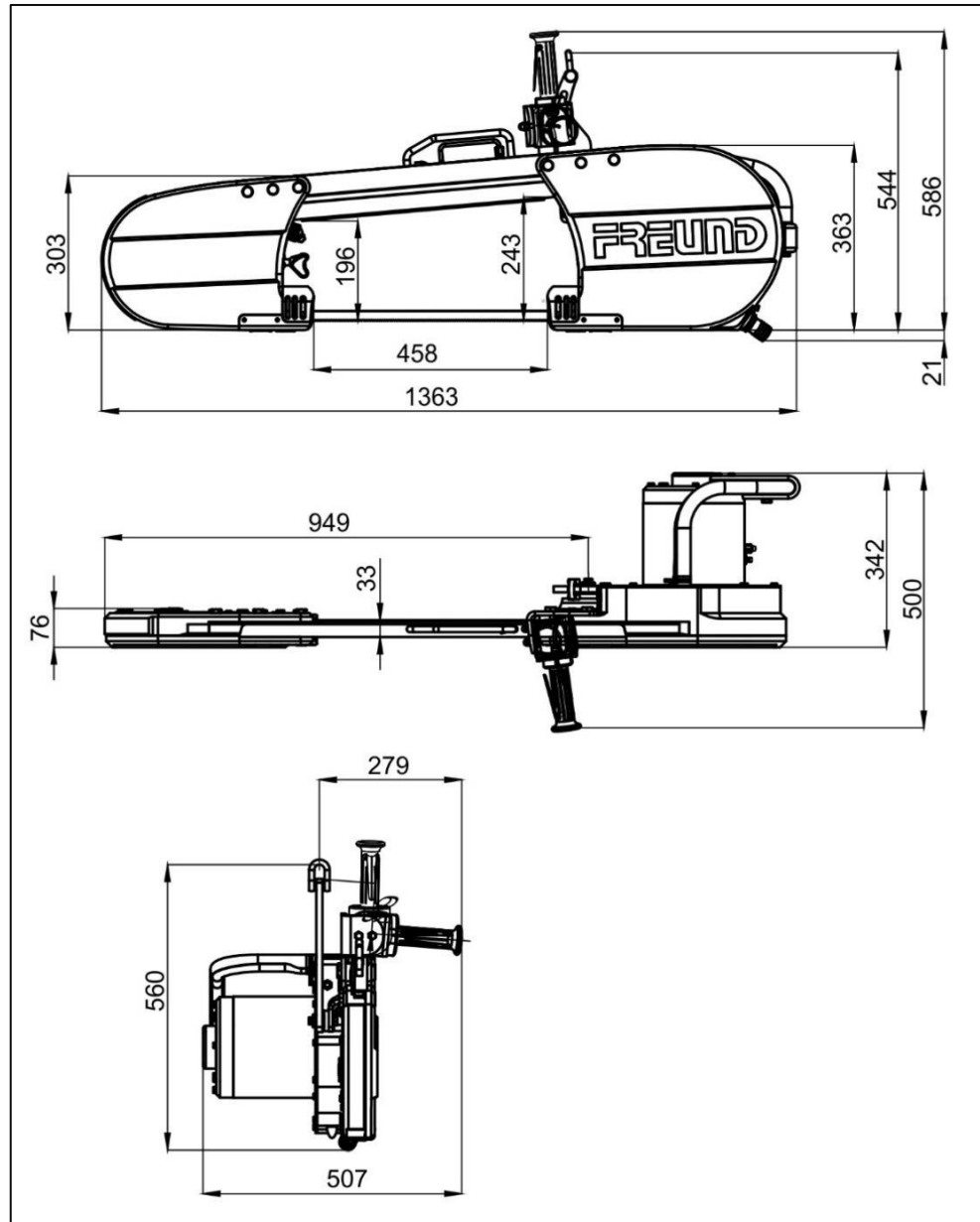
Fig. 3-3 Dimensiones de la sierra de cinta de esquinado [datos en mm]
