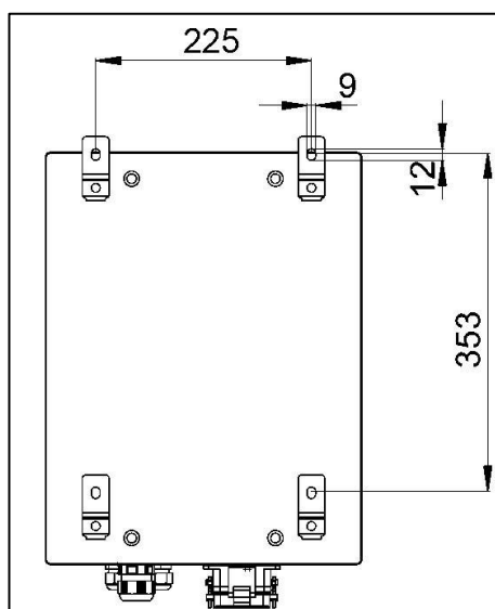
Fig. 5-2 Gráfico de agujeros del dispositivo interruptor [datos en mm]
