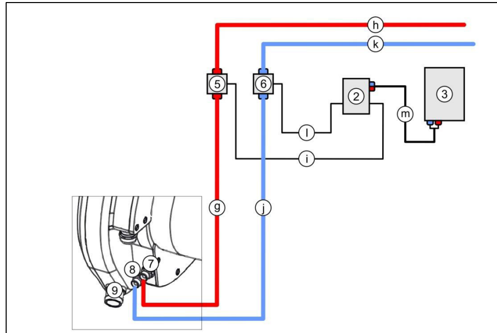
Fig. 5-7 Esquema de conexión con caja de distribución (opcional)
