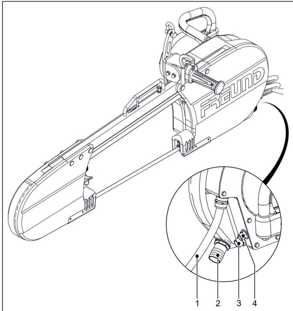
Abb. 3-2 Position der Anschlüsse
