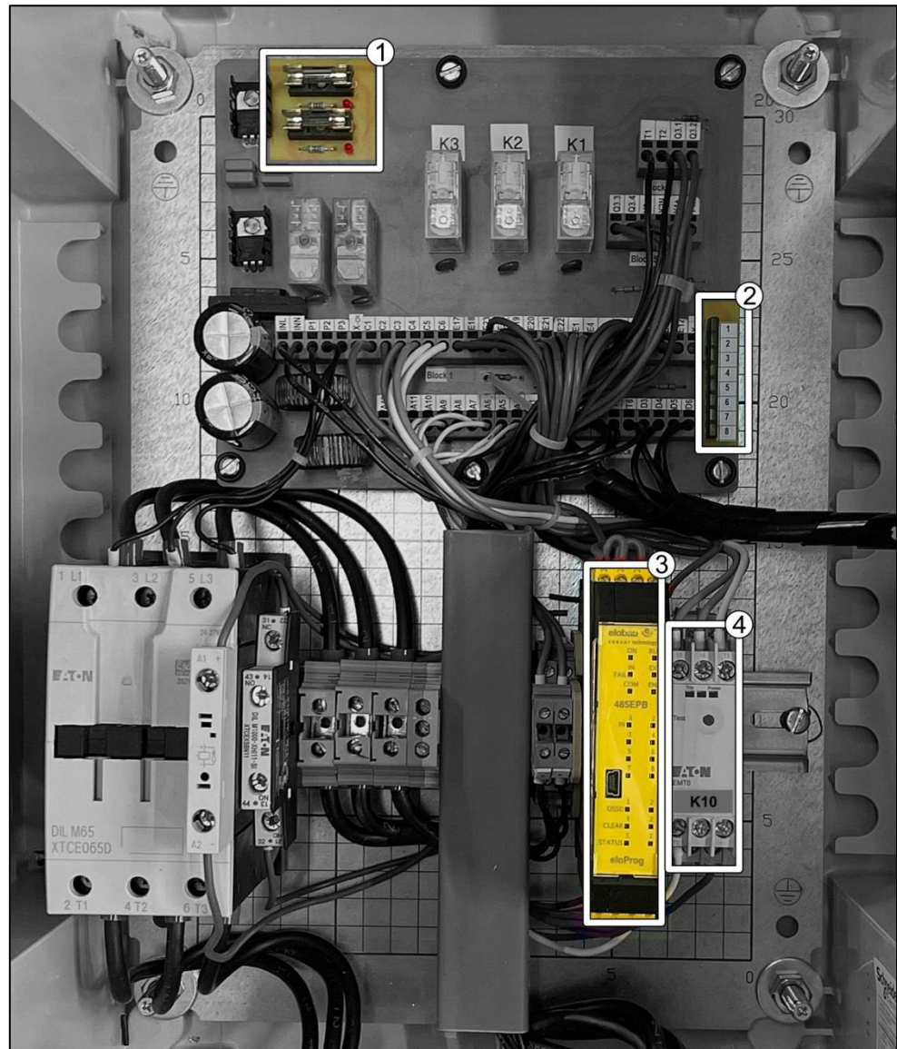
Abb. 9-1 LED-Statusanzeigen im Schaltgerät
