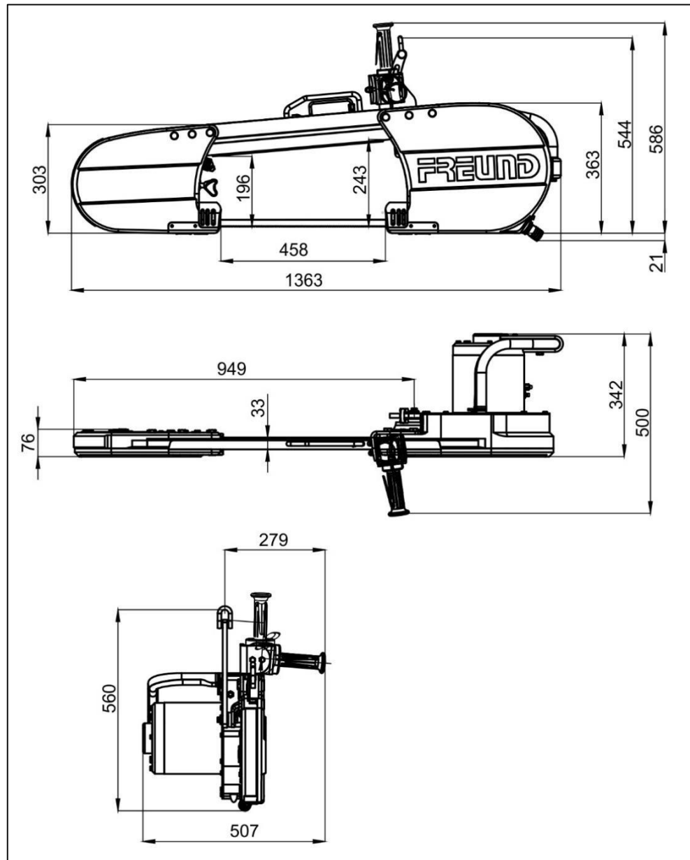
Abb. 3-3 Abmessungen Spalt-Bandsäge (Angaben in mm)
