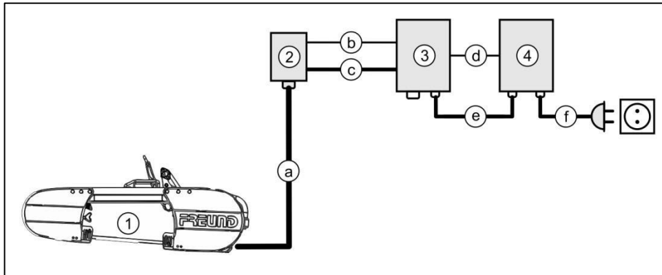
Abb. 5-5 Anschlusschema mit Verteilerbox (optional)
