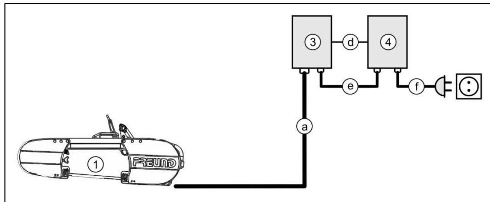
Abb. 5-4 Anschlusschema
