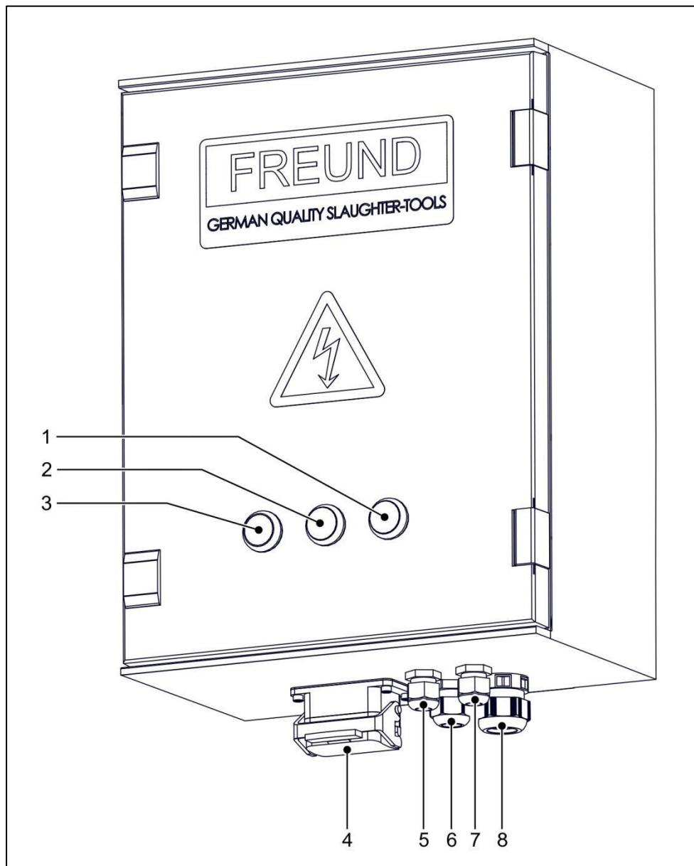
Abb. 3-4 Ansicht Schaltgerät SG SB46-24
