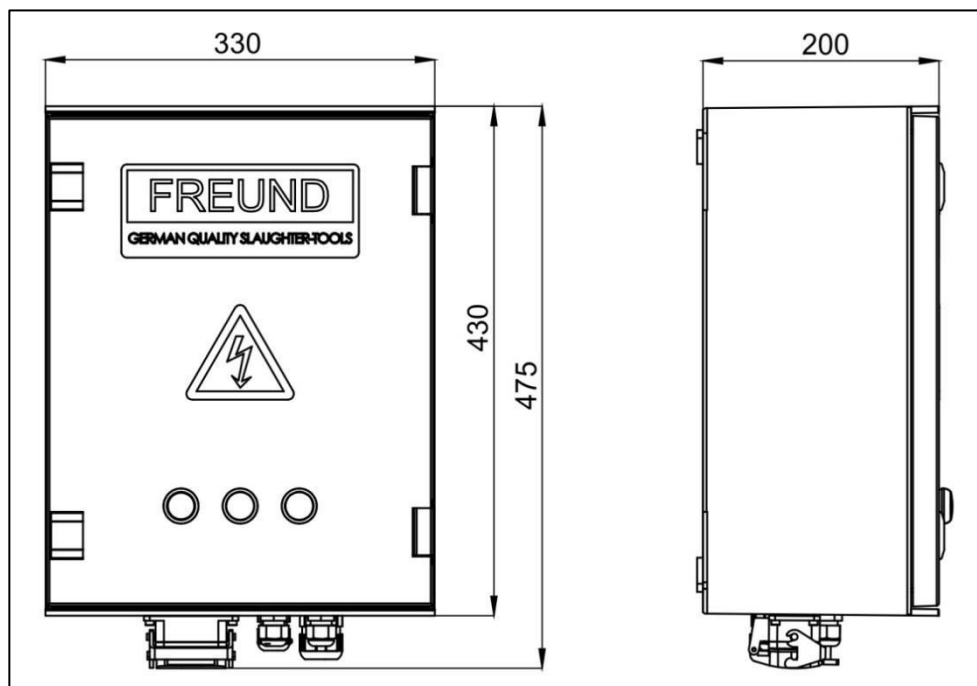
Abb. 3-5 Abmessungen Schaltgerät (Angaben in mm)
