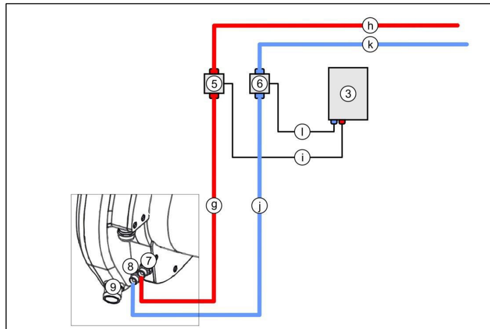
Abb. 5-6 Anschlussschema
