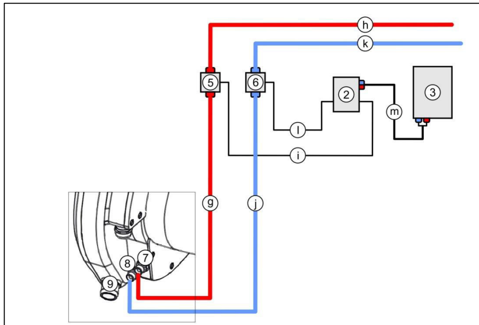
Pos. Beschreibung 2 Verteilerbox (optional): Verlängerung der Anschlussleitungen bei großen Distanzen zwischen Spalt-Bandsäge und Schaltgerät m Steuerungskabel Magnetventile „Innendesinfektion“ und „Kühlung“: Verteilerbox <> Schaltgerät 3 Schaltgerät SG SB46-24 5 Magnetventil für Funktion „Innendesinfektion“ g Wasserschlauch „Innendesinfektion“: Spalt-Bandsäge <> Magnetventil h Wasserschlauch „Innendesinfektion“: Magnetventil <> bauseitiger Anschluss i Steuerungskabel Magnetventil „Innendesinfektion“: Magnetventil <> Verteilerbox 6 Magnetventil für Funktion „Kühlung“ j Wasserschlauch „Kühlung“: Spalt-Bandsäge <> Magnetventil k Wasserschlauch „Kühlung“: Magnetventil <> bauseitiger Anschluss l Steuerungskabel Magnetventil „Kühlung“: Magnetventil <> Verteilerbox 7 Anschluss „Innendesinfektion“ an der Spalt-Bandsäge 8 Anschluss „Kühlung“ an der Spalt-Bandsäge 9 Wasserabfluss an der Spalt-Bandsäge
