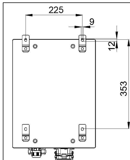
Abb. 5-2 Bohrbild Schaltgerät [Angaben in mm]
