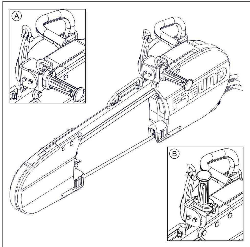
Abb. 3-1 Ansicht SB46-24 mit Details zur einstellbaren Ausrichtung des Handgriffs (A), (B)
