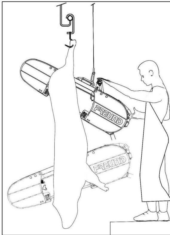
Abb. 6-1 Maschine bedienen
