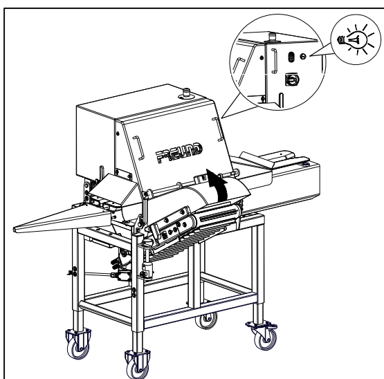
Fig. 6-2 Contrôle du capot de protection du convoyeur
