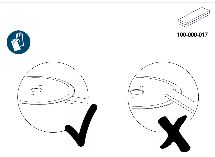
Fig. 8-1 Affûtage du couteau circulaire
