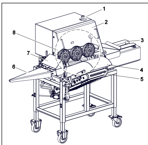
Fig. 3-1 Vue avant de la machine
