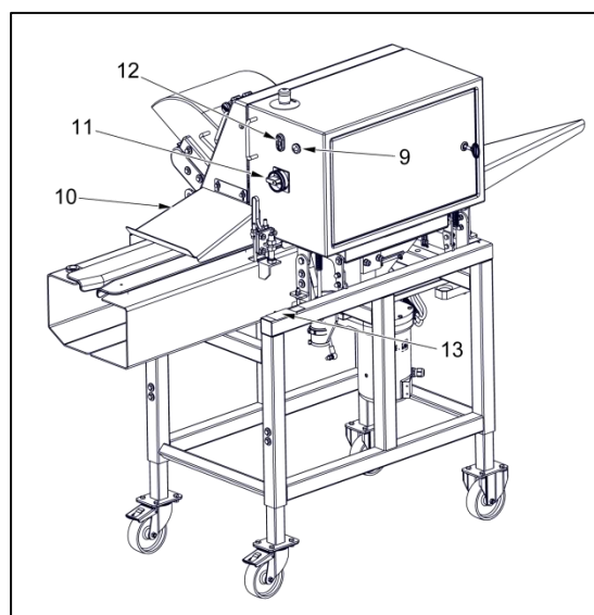
Fig. 3-2 Vue arrière de la machine
