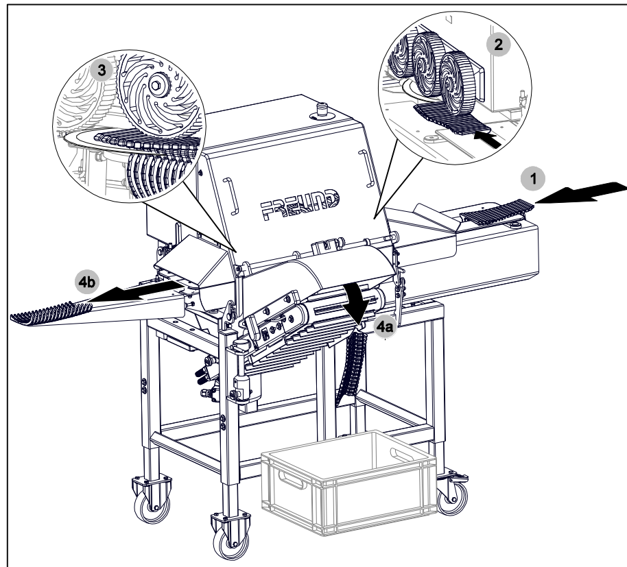
Fig. 6-5 Commande de la machine
