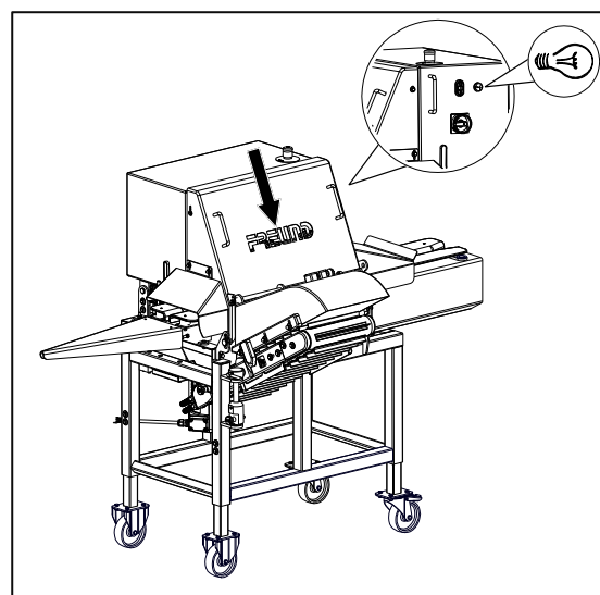
Fig. 6-1 Contrôle du capot de protection du galet de transport
