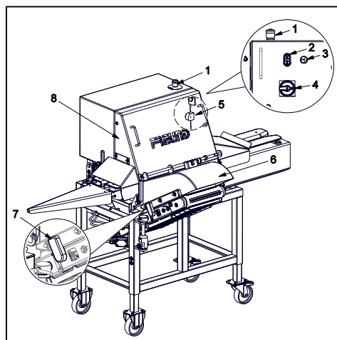
Fig. 2-2 Positionnement des dispositifs de sécurité
