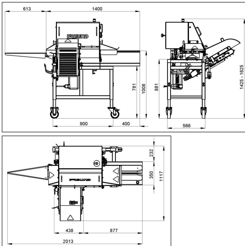
Fig. 3-3 Dimensions SRC [données en mm]
