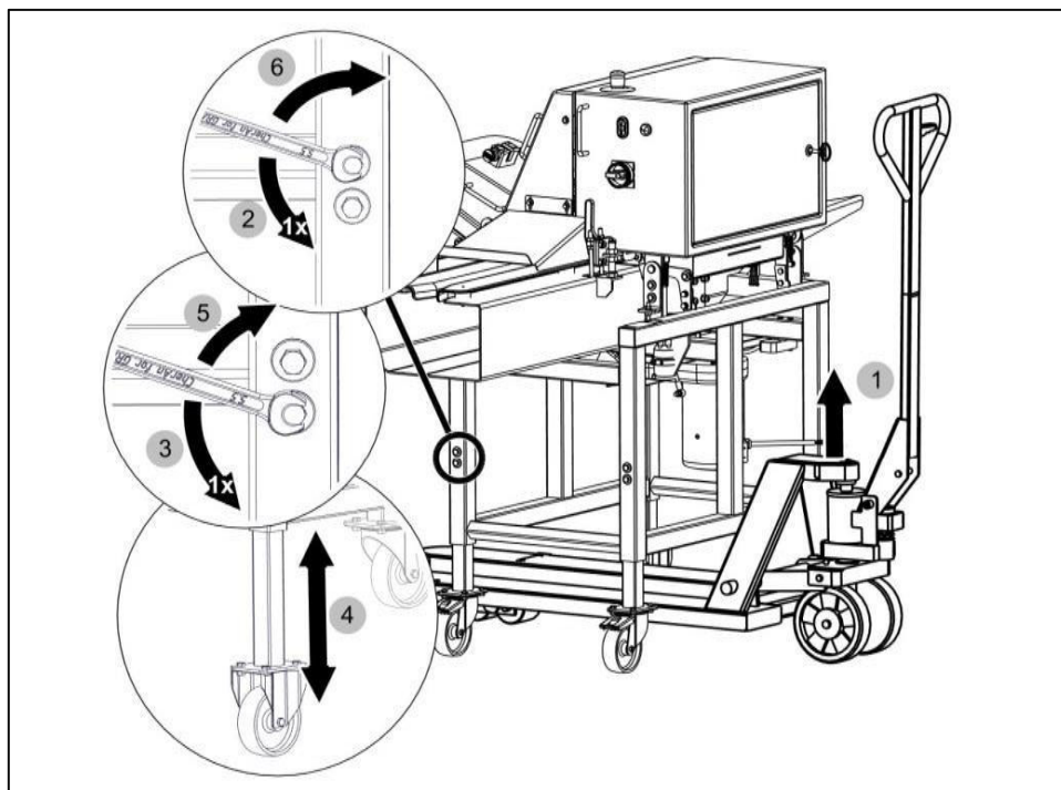
Fig. 5-1 Procédure de modification de la hauteur de travail
