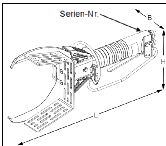
Afb. Schaar model HDS15
