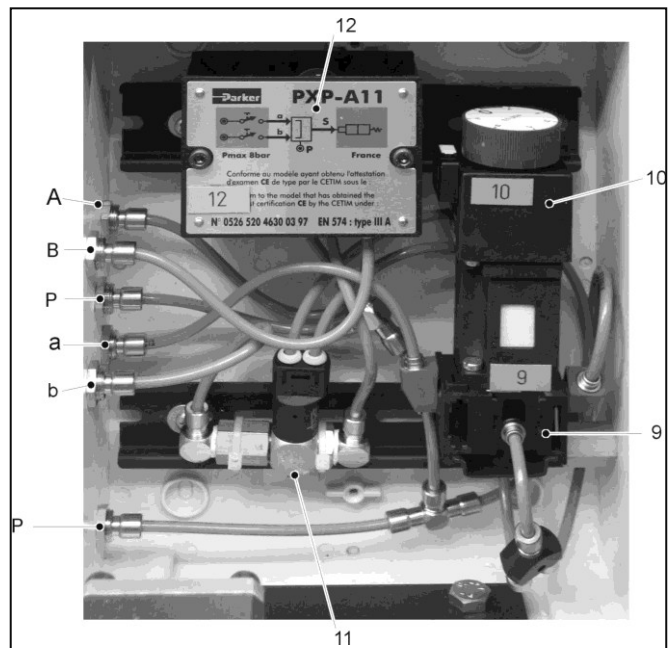
Afb. 3-6 Schakelkast binnenzijde
