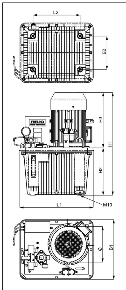
Afb. Afmetingen HPE9 / HPE20
