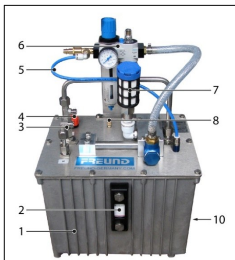
Afb. Aanzicht HPP12
