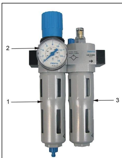
Ilust. 3-11 Unidad de mantenimiento
