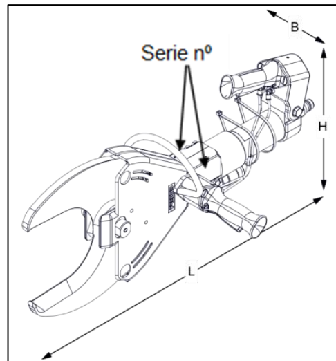
Fig. Cizalla modelo LS15
