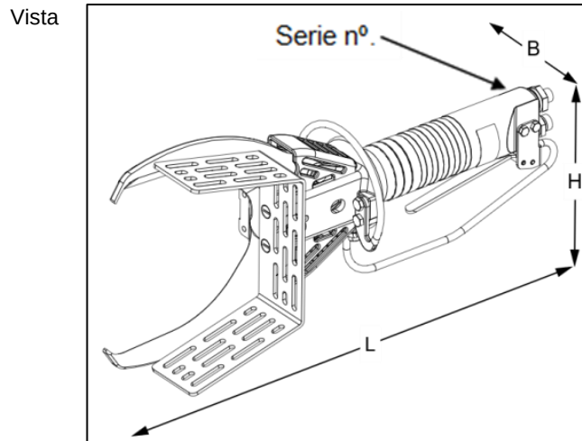
Fig. Cizalla modelo HDS15
