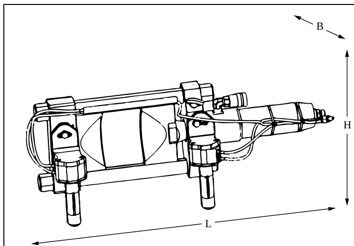
Imag. 3-8 Guillotina de descorne HG12 evo2
