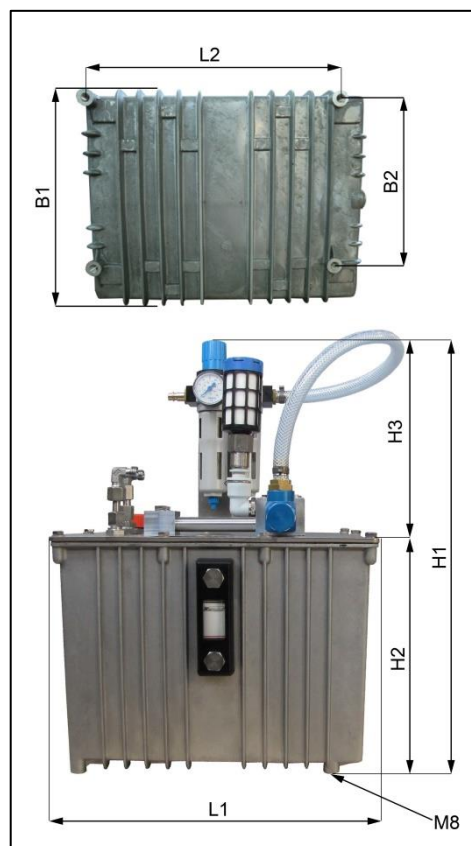
Fig. 3-9 Dimensiones HPP12
