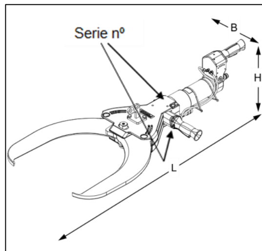
Fig. Cizalla modelo AS28
