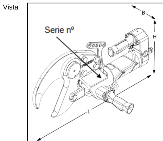
Fig. Cizalla modelo HLS12
