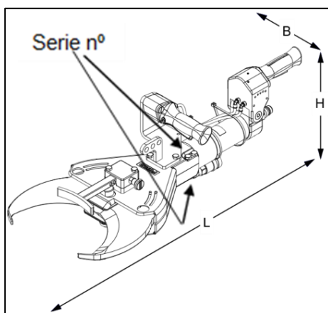
Fig. 3-5 Cizalla modelo NS21
