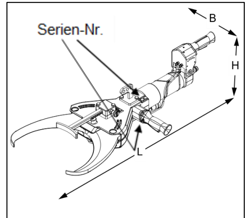
Abb. 3-9 Schere Model NS26
