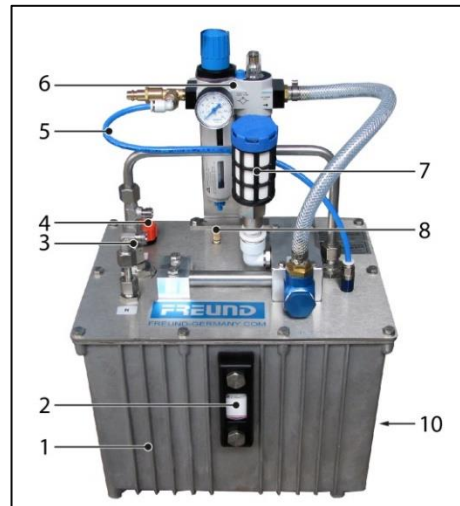
Abb. 3-13 Ansicht HPP12
