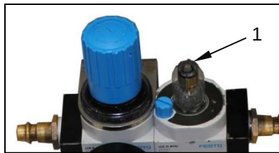
Abb. 5-2 Wartungseinheit befüllen
