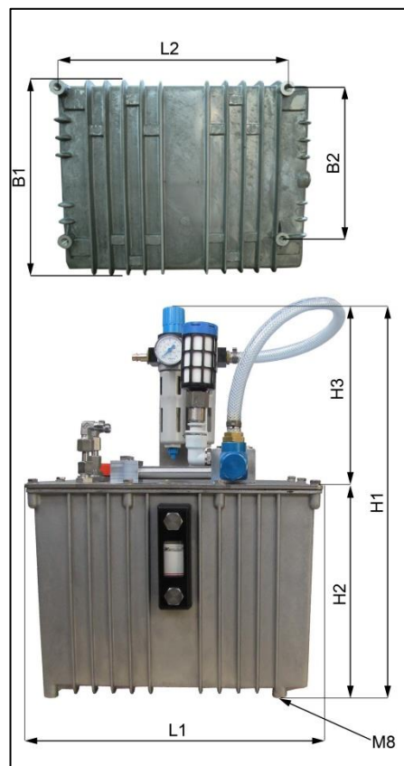
Abb. 3-15 Abmessungen HPP12
