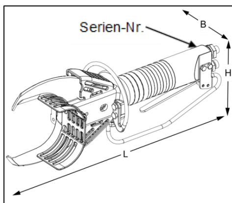
Abb. 3-3 Abbildungsbeispiel für FNS9 mit Bügel und vertikalem Messer
