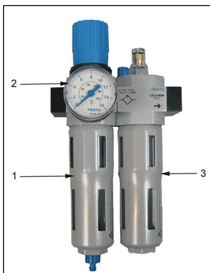
Abb. 3-20 Wartungseinheit
