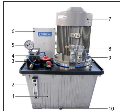
Abb. 3-14 Ansicht HPE20
