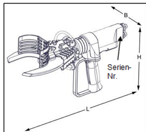
Abb. 3-4 Abbildungsbeispiel für FNS9 mit Pistolenhandgriff und horizontalem Messer
