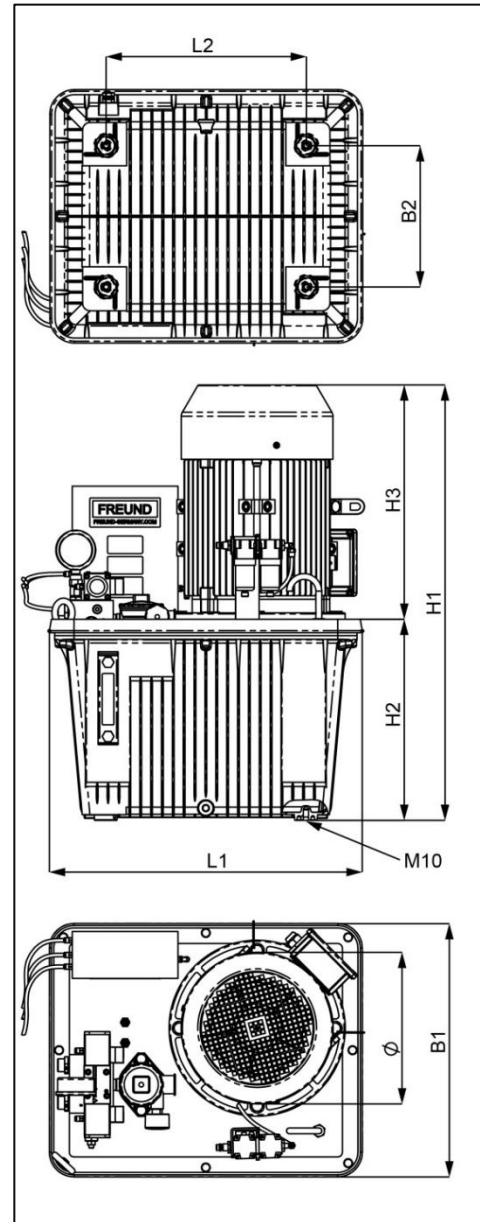
Abb. 3-16 Abmessungen HPE9 / HPE20
