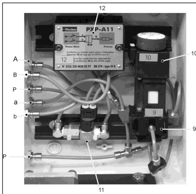
Abb. 3-19 Schaltkasten innen
