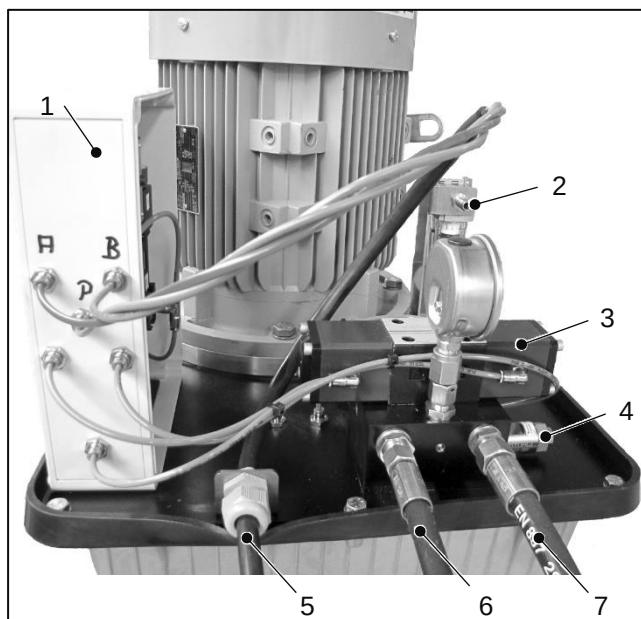
Abb. 3-17 Elektrische Steuerelemente
