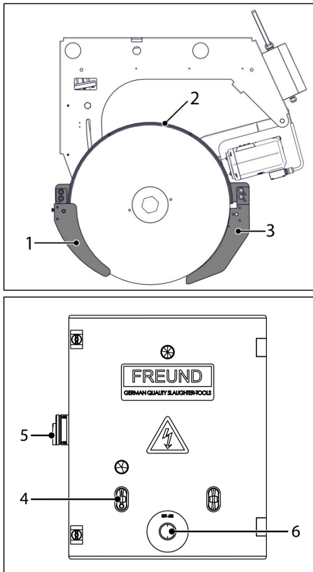
Fig. 2-1 Éléments de sécurité ZKM
