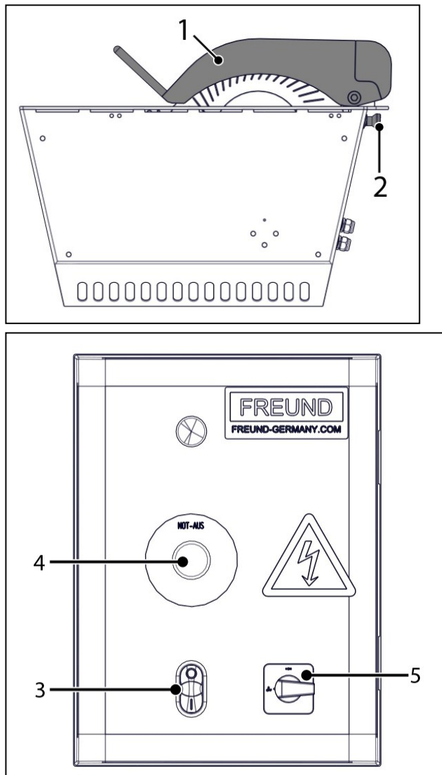
Fig. 2-4 Éléments de sécurité FK40
