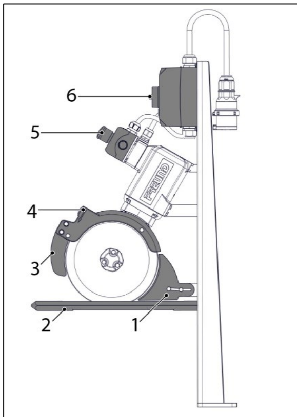
Fig. 2-3 Éléments de sécurité ZKM25
