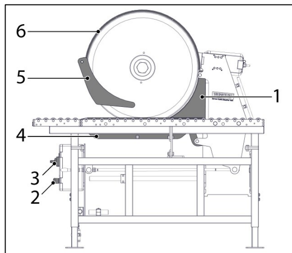
Fig. 2-2 Éléments de sécurité ZKM (version pour table)
