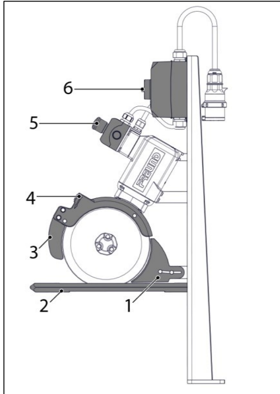
Abb. 2-3 Sicherheitselemente ZKM25
