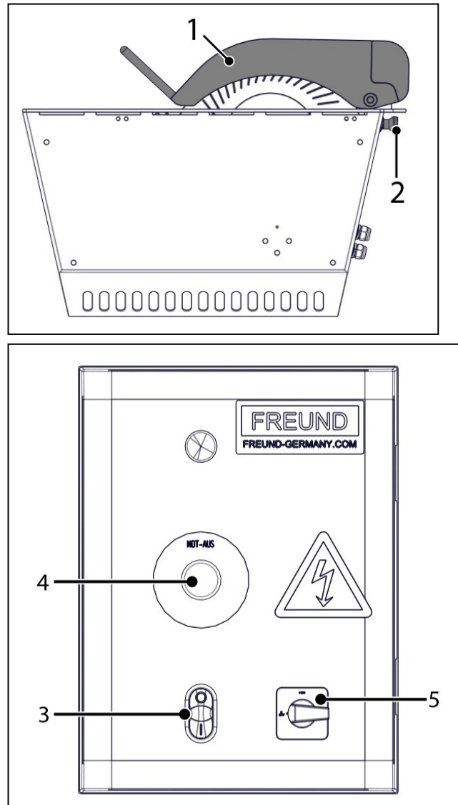
Abb. 2-4 Sicherheitselemente FK40
