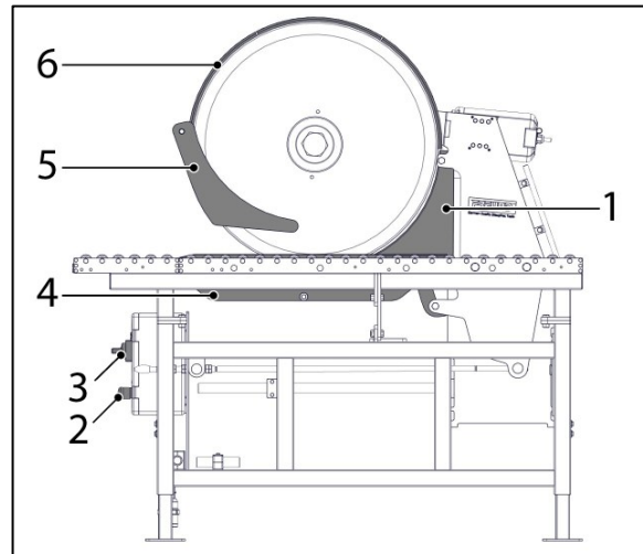
Abb. 2-2 Sicherheitselemente ZKM (Tischversion)
