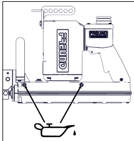
Abb. 8-1 Lage der Schmiernippel
