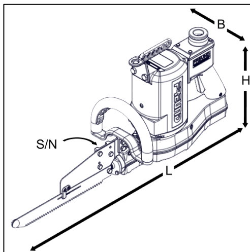
Abb. 3-4 Beispielabbildung Brustbein-Stichsäge
