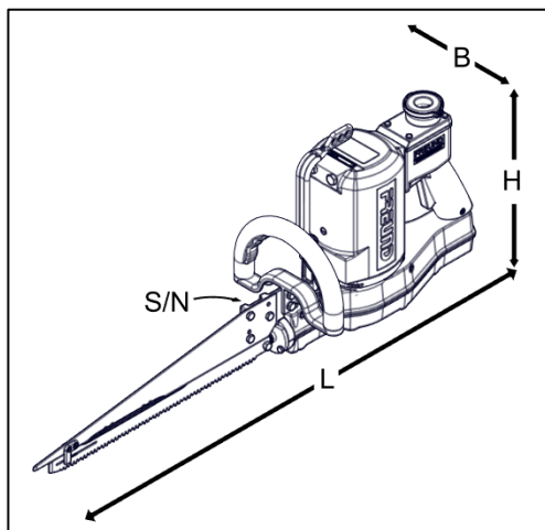
Abb. 3-6 Zerlege-Stichsäge
