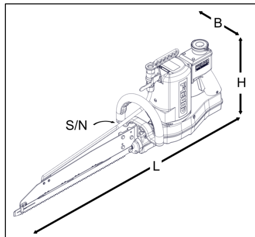
Abb. 3-5 Beispielabbildung Spalt-Stichsäge
