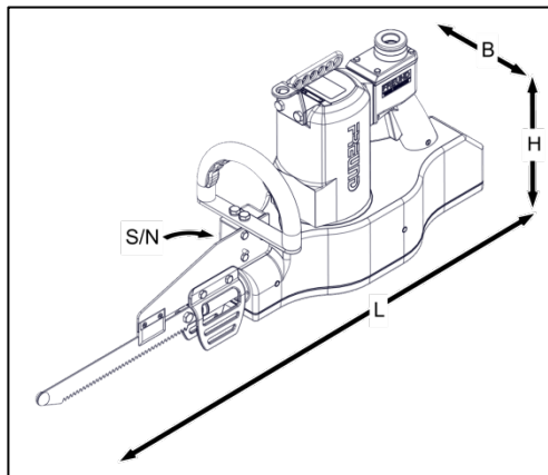
Abb. 3-2 Beispielabbildung Brustbein-Hubsäge
