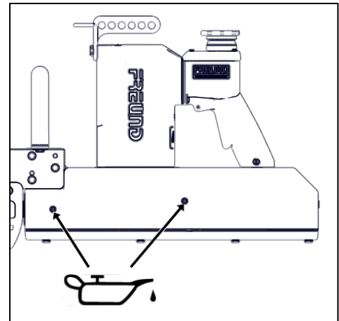
Abb. 8-1 Lage der Schmiernippel
