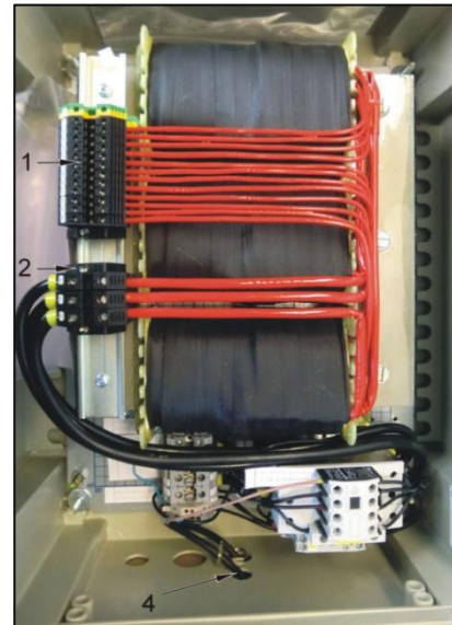
Afb. 5-9 Inwendige aansluitingen TR7
