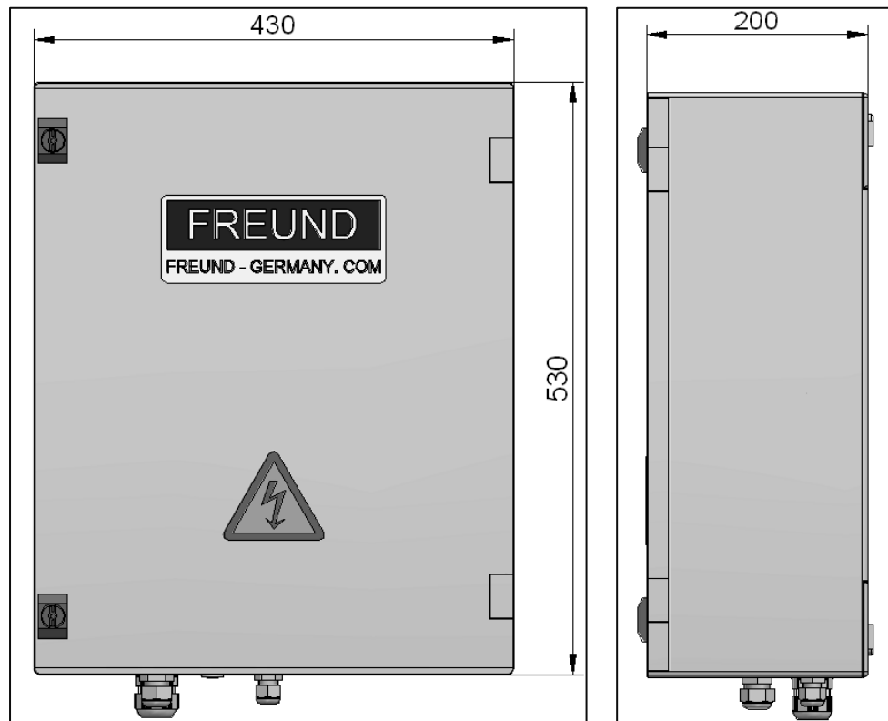
Fig. 3-1 – Fig. 3-2 Dimensions
