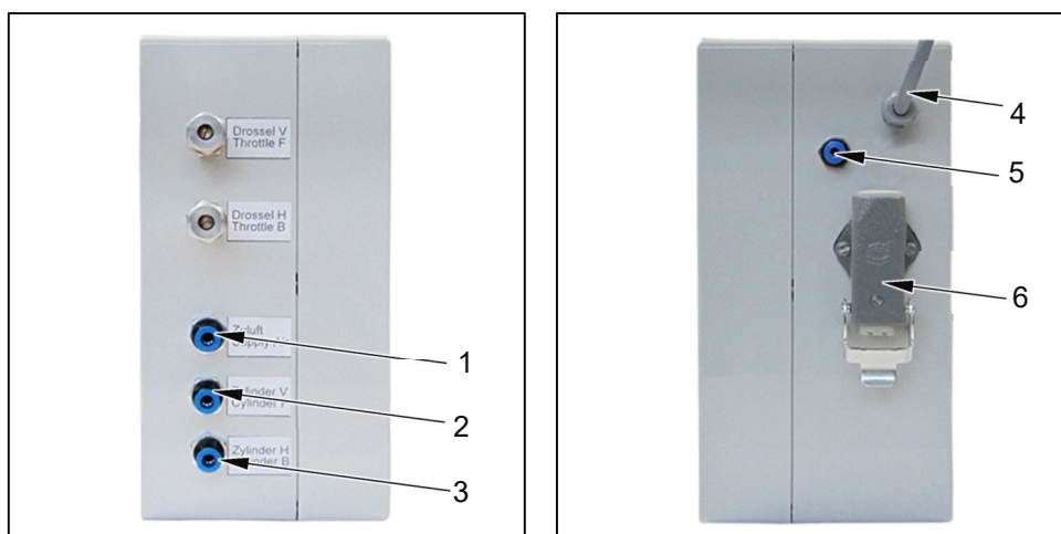
Рис. 3-10 Присоединительные элементы (интерфейсный блок управления: версия с 1 цилиндром)
