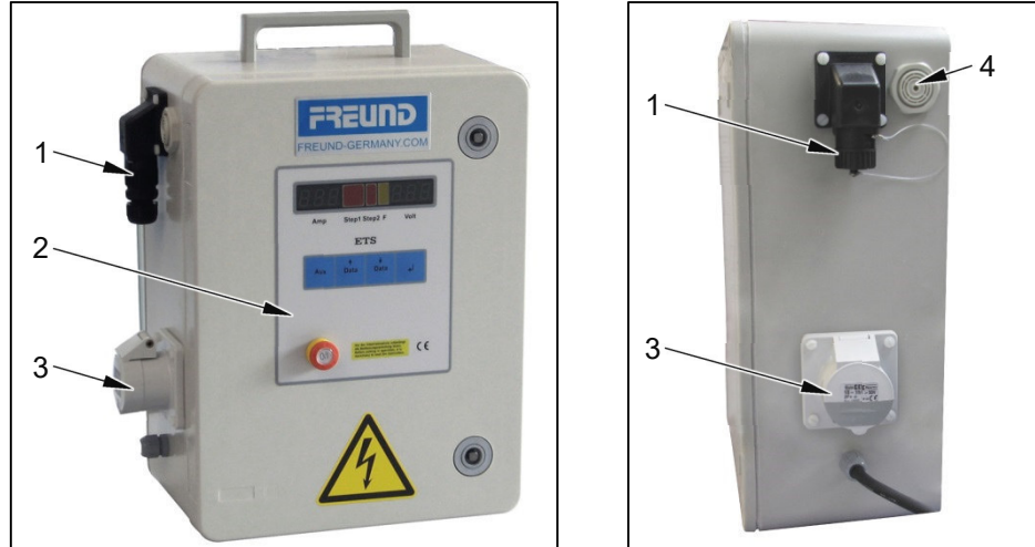
Рис. 3-1 Функциональные узлы
