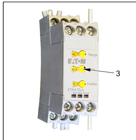
Afb. 3-12 Tijdrelais
