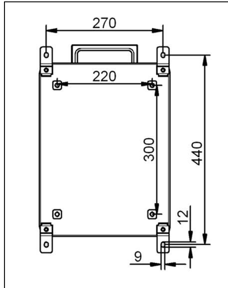
Afb. 5-4 Maten boorsjabloon
