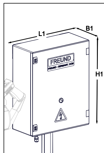
Рис. 3-8 Пример изображения коммутационного аппарата
