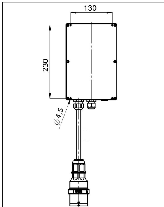
Fig. 5-14 Control box hole pattern 2HADTS 400 V
