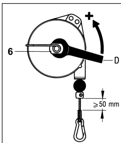
Рис. 5-2 Увеличение грузоподъемности
