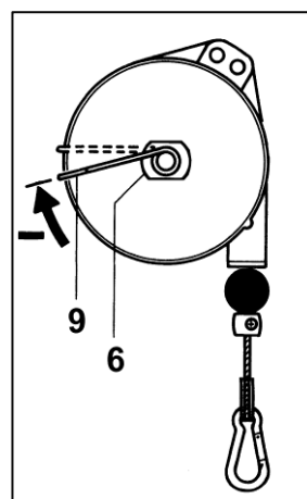
Рис. 5-3 Уменьшение грузоподъемности
