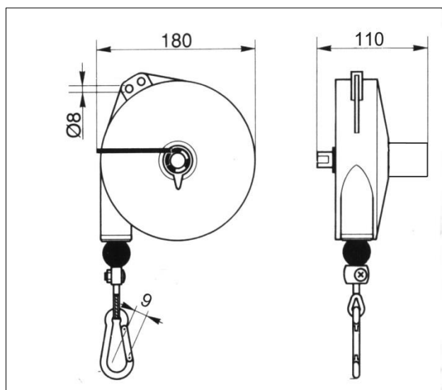
Рис. 3-1 Размеры
