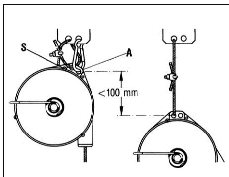
Рис. 4-3 Основное подвесное устройство пружинного балансира
