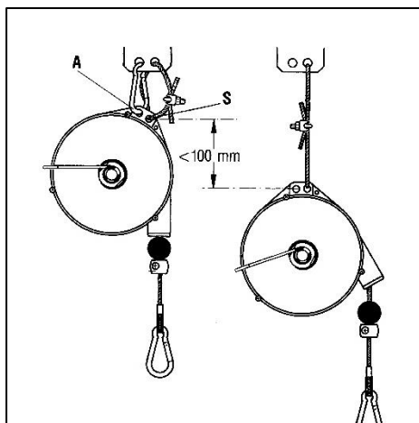
Рис. 4-1 Основное подвесное устройство пружинного балансира
