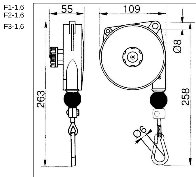
Рис. 3-1 Размеры
