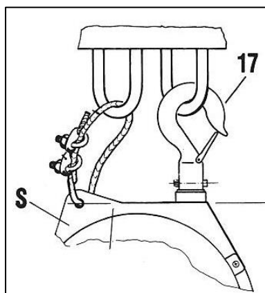
Рис. 4-3 Страховочное подвесное устройство
