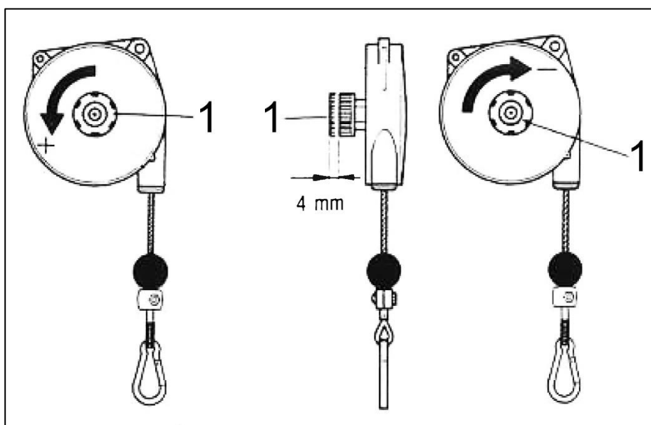
Рис. 5-2 Регулировка грузоподъемности
