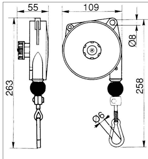
Abb. 3-1 Abmessungen
