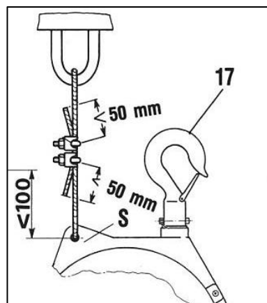
Abb. 4-1 Fallhöhe
