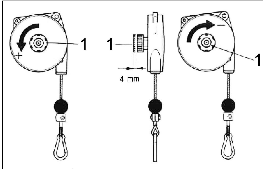
Abb. 5-2 Tragleistung einstellen
