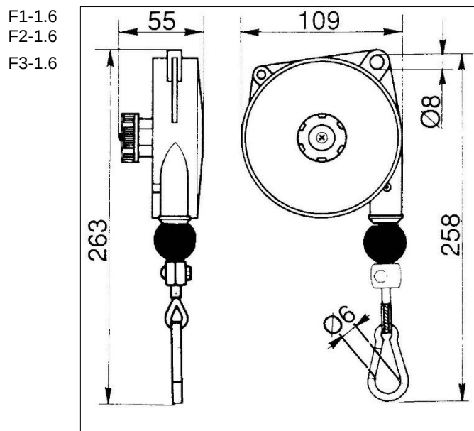
Fig. 3-1 Dimensions
