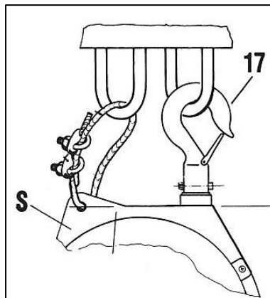
Abb. 4-3 Sicherheitsaufhängung
