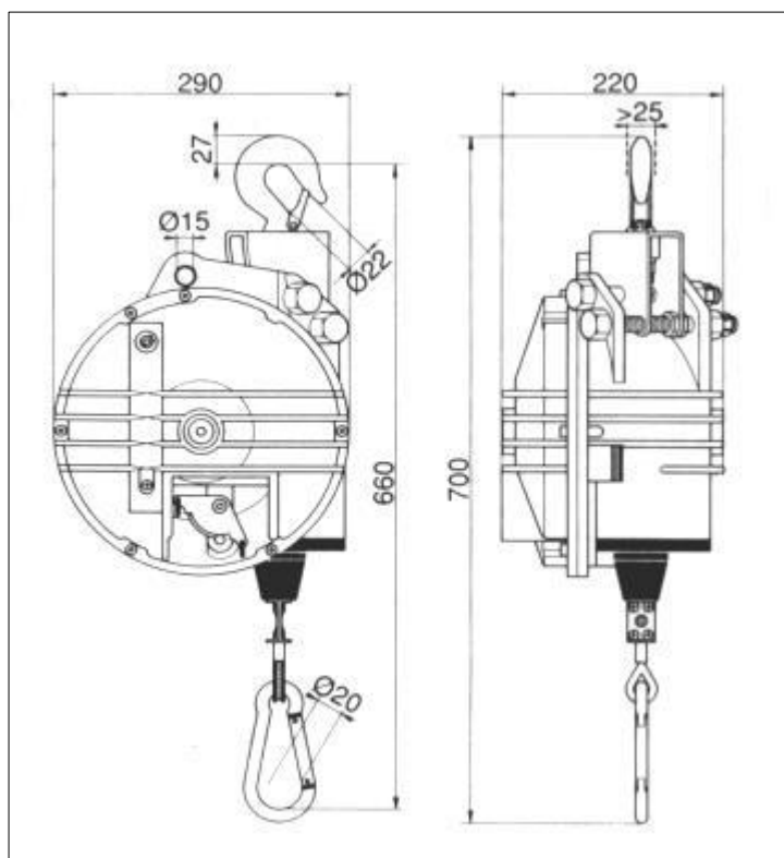
Рис.3-1 Размеры пружинных балансиров F20-F35
