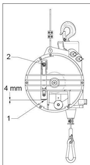
Рис. 5-3 Зажимной винт
