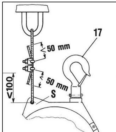
Abb. 4-1 Fallhöhe
