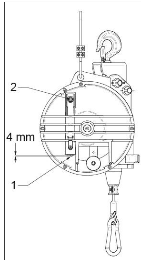
Abb. 5-3 Spannschraube
