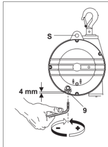
Abb. 5-2 Tragleistung einstellen
