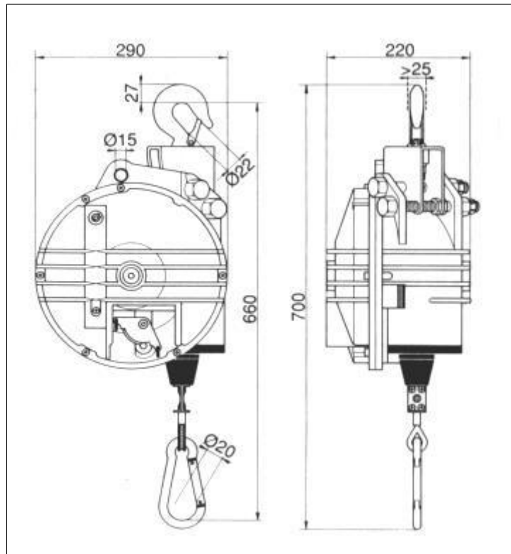
Abb.3-1 Abmessungen Federzüge F20-F35
