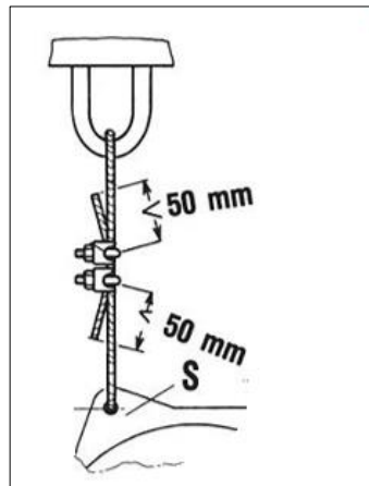
Abb. 4-4 Montage Sicherungsseil
