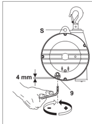
Abb. 5-2 Tragleistung einstellen
