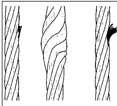
Abb. 6-1 Sichtbare Schäden am Seil
