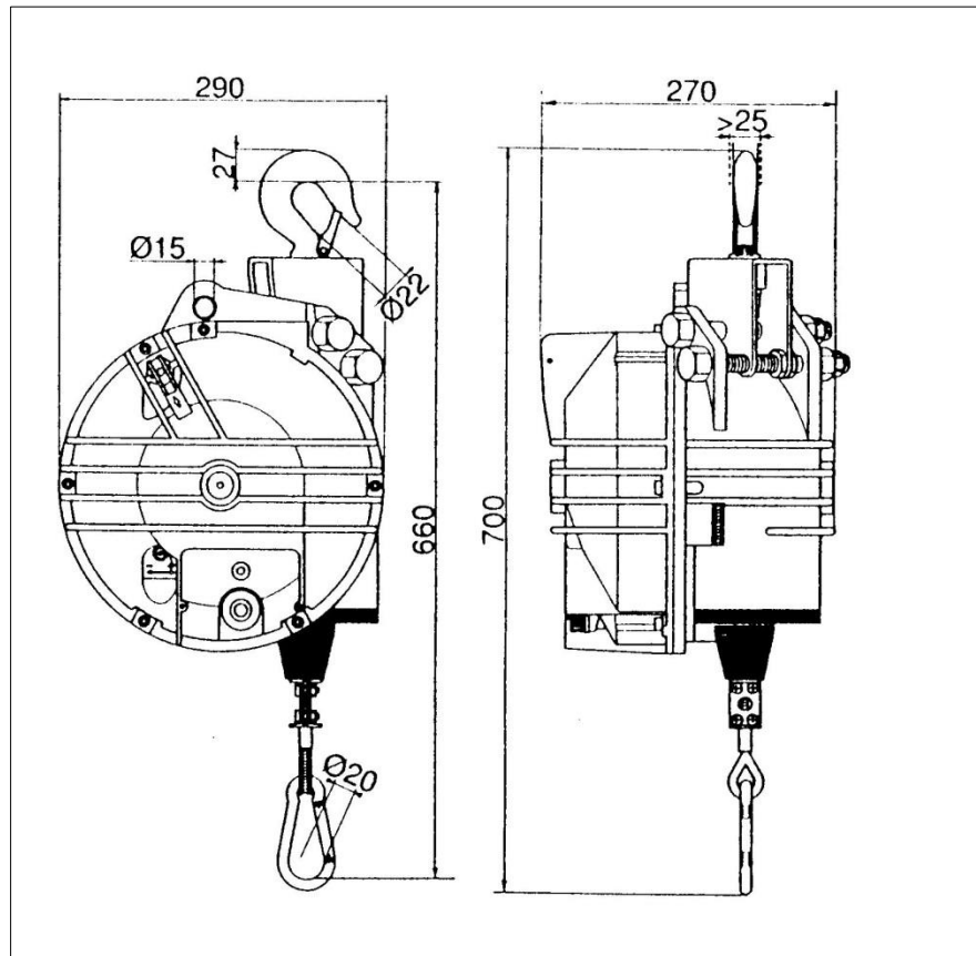
Fig. 3-1 Dimensions
