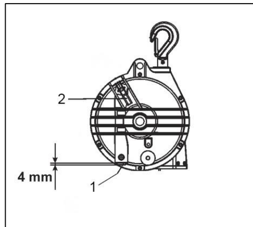
Abb. 5-3 Spannschraube
