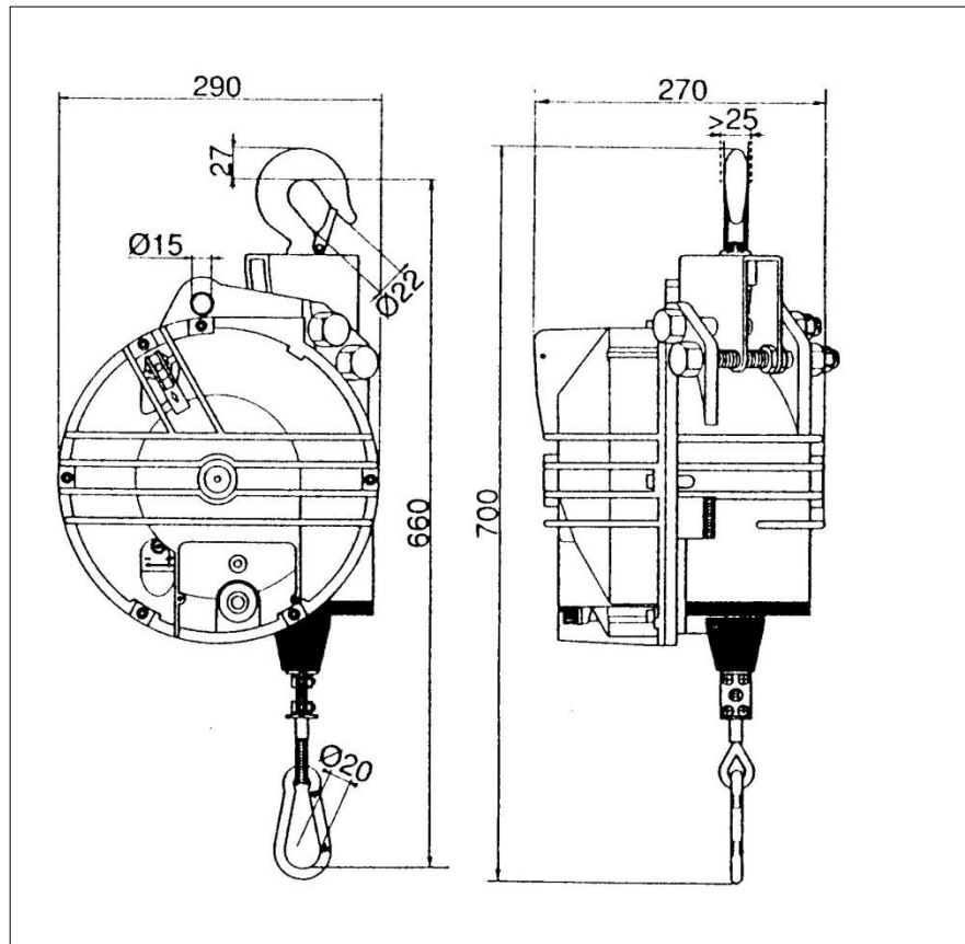
Abb. 3-1 Abmessungen
