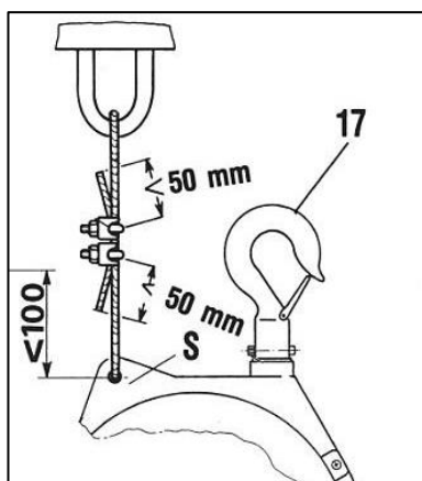
Рис. 4-1 Высота падения
