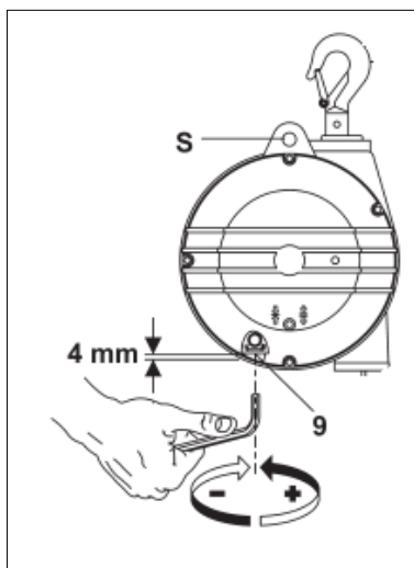
Рис. 5-2 Регулировка грузоподъемности
