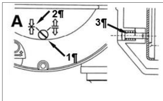
Рис. 5-4 Блокировка барабана
