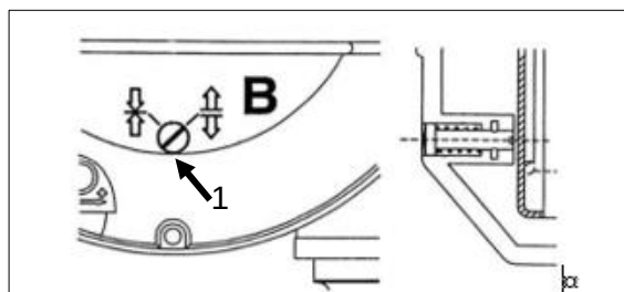
Рис. 5-3 Свободное положение установочного винта
