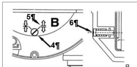
Abb. 5-5 Trommel freigeben
