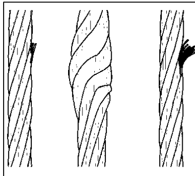
Abb. 6-1 Sichtbare Schäden am Seil
