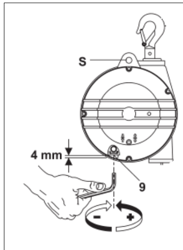
Abb. 5-2 Tragleistung einstellen
