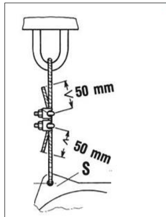
Abb. 4-4 Montage Sicherungsseil
