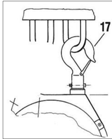
Abb. 4-2 Federzug aufhängen
