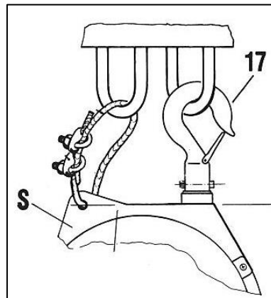
Abb. 4-3 Sicherheitsaufhängung
