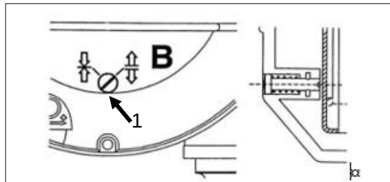
Abb. 5-3 Geöffnete Stellung Einstellschraube
