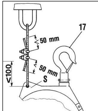
Abb. 4-1 Fallhöhe
