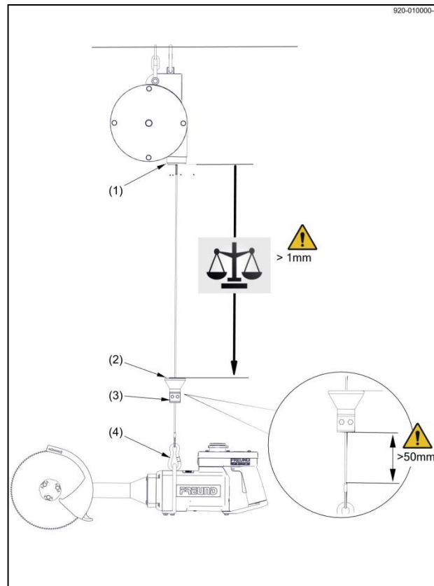
Abb. 5-1 Angehängte Kreissäge
