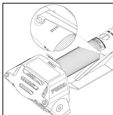
Fig. 3-7 Número de serie de cinco cifras
