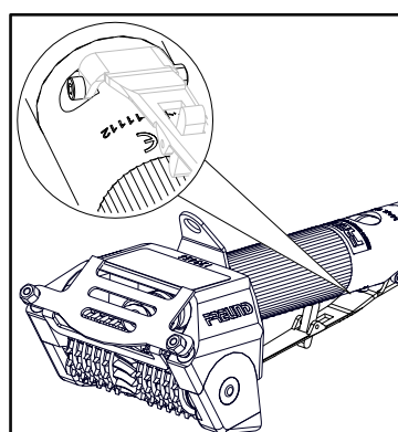
Ilust. 3-9 Número de serie de cinco cifras
