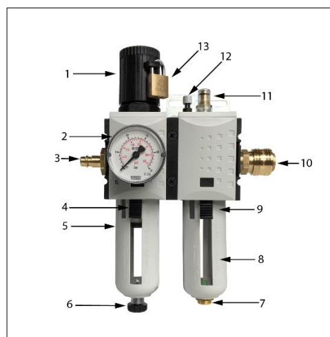
Fig. 4-1 Unidad de mantenimiento
