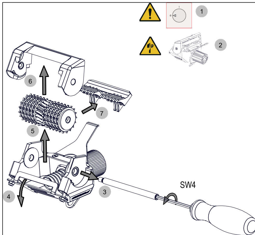
Fig. 6-1 Limpieza de la máquina
