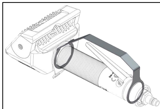
Abb. 2-1 Schutzbügel (dunkel hervorgehoben)
