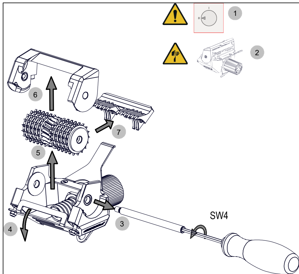
Abb. 6-1 Maschine reinigen
