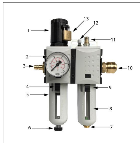
Abb. 4-1 Wartungseinheit
