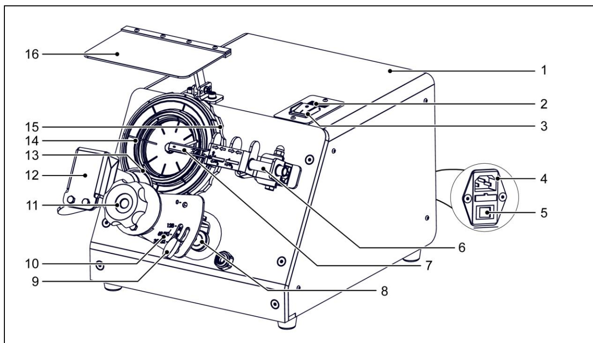
Afb. 3-13 Aanzicht TSM-E1
