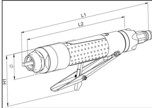
Afb. 3-9 Afmetingen pneumatische motor P2
