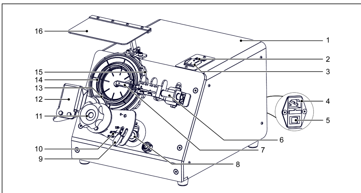
Fig. 3-13 Vue TSM-E1
