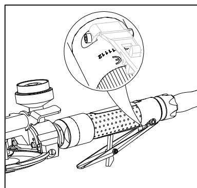
Fig. 3-10 N° de série à 6 chiffres du moteur P2
