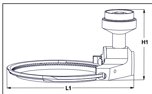
Fig. 3-1 Vue latérale
