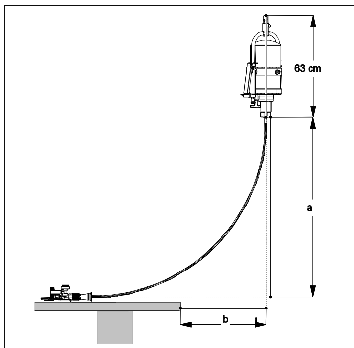
Fig. 5-1 Schéma de positionnement du moteur électrique
