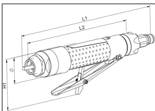
Fig. 3-9 Dimensions du moteur pneumatique P2
