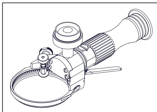
Fig. 3-7 Trimmer électrique avec entraînement Start/Stop
