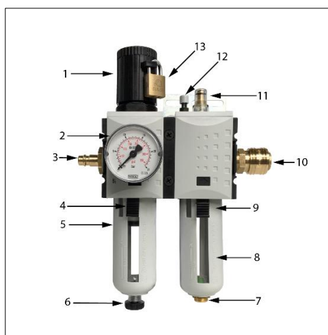
Fig. 3-12 Unité de maintenance
