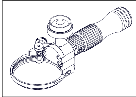
Fig. 3-6 Trimmer électrique avec entraînement permanent
