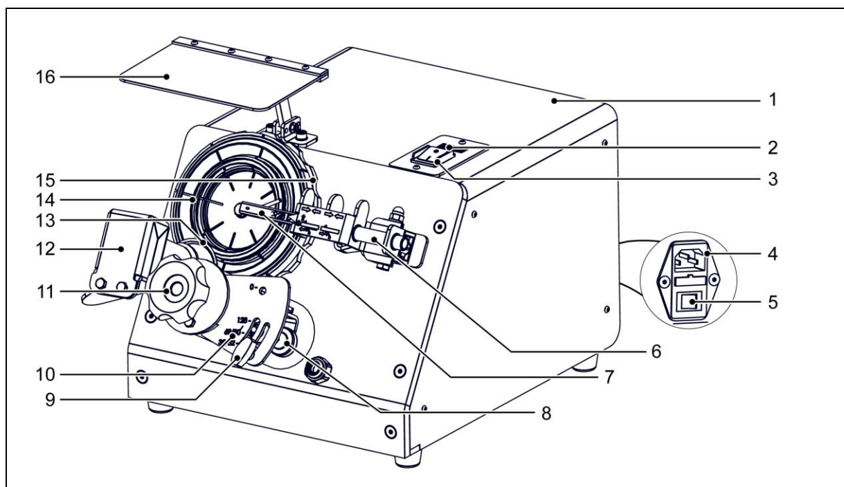
Imag. 3-13 Vista TSM E1
