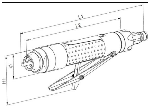
Ilust. 3-9 Dimensiones motor neumático P2
