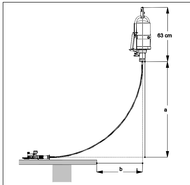
Ilust. 5-1 Esquema de posicionamiento para el motor eléctrico
