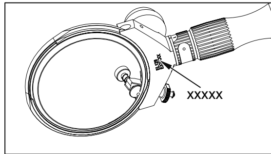
Ilust. 3-3 Número de serie de cinco cifras del cabezal del cuchillo circular
