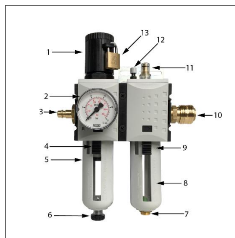
Fig. 3-12 Unidad de mantenimiento
